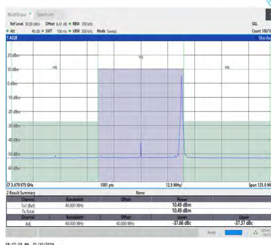
NTNV_N48_30_40_H_TID18_#1_-40_40
