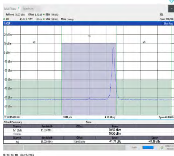
NTNV_N48_30_15_H_TID18_#1_-15_15
