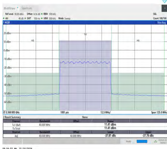
NTNV_N48_30_40_L_TID16_#1_-40_40
