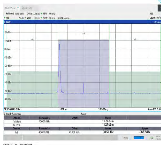
NTNV_N48_30_40_L_TID17_#1_-40_40
