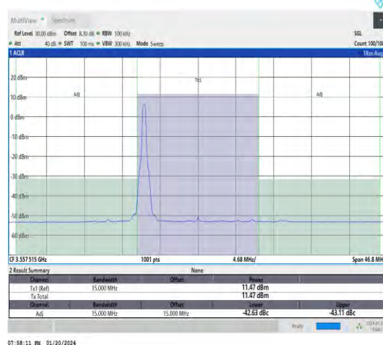
NTNV_N48_30_15_L_TID17_#1_-15_15
