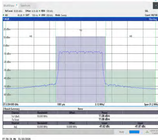
NTNV_N48_30_10_L_TID16_#1_-10_10
