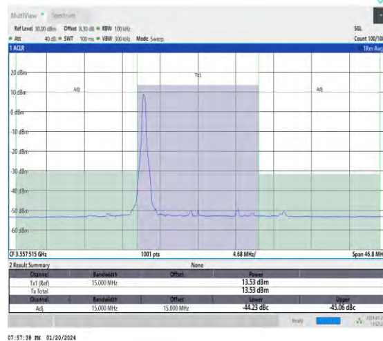
NTNV_N48_30_15_L_TID2_#1_-15_15
