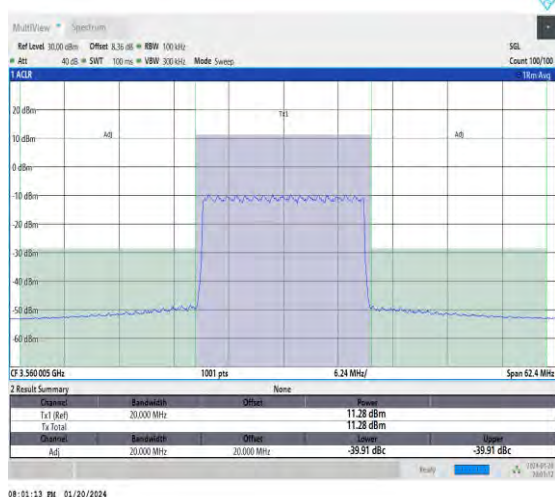
NTNV_N48_30_20_L_TID16_#1_-20_20
