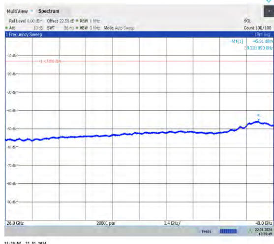
NTVN_N48_30_40_L_TID1_NS_01_26000_40000_#1
