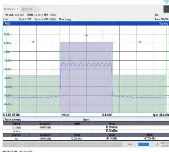
NTNV_N48_30_40_H_TID16_#1_-40_40
