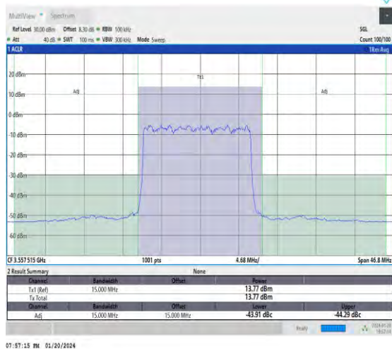
NTNV_N48_30_15_L_TID1_#1_-15_15
