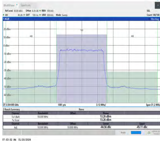
NTNV_N48_30_10_L_TID1_#1_-10_10
