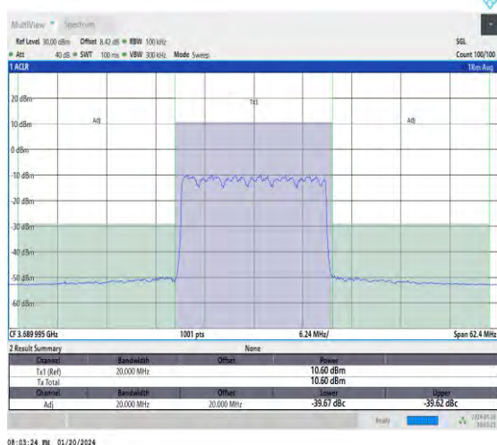
NTNV_N48_30_20_H_TID16_#1_-20_20
