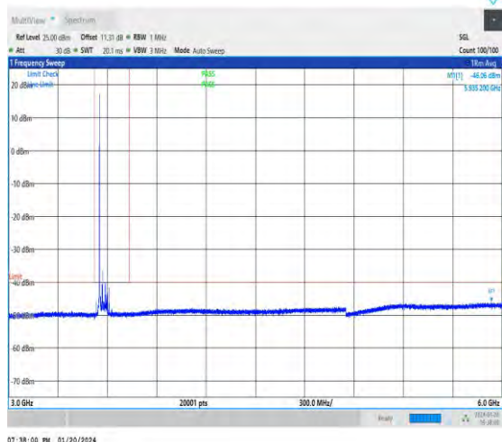
NTVN_N48_30_40_L_TID1_NS_01_3000_6000_#1
