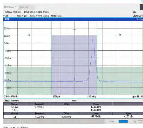
NTNV_N48_30_10_H_TID18_#1_-10_10
