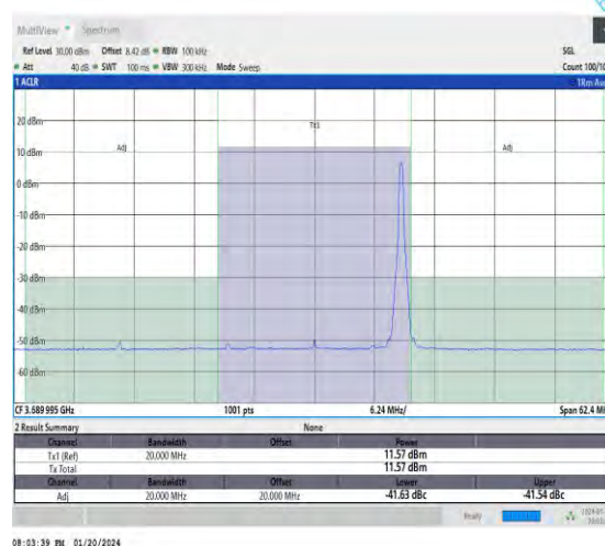
NTNV_N48_30_20_H_TID18_#1_-20_20
