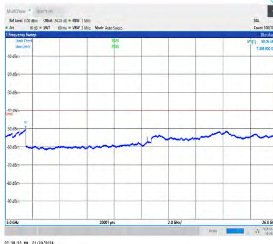
NTVN_N48_30_40_L_TID1_NS_01_6000_26000_#1
