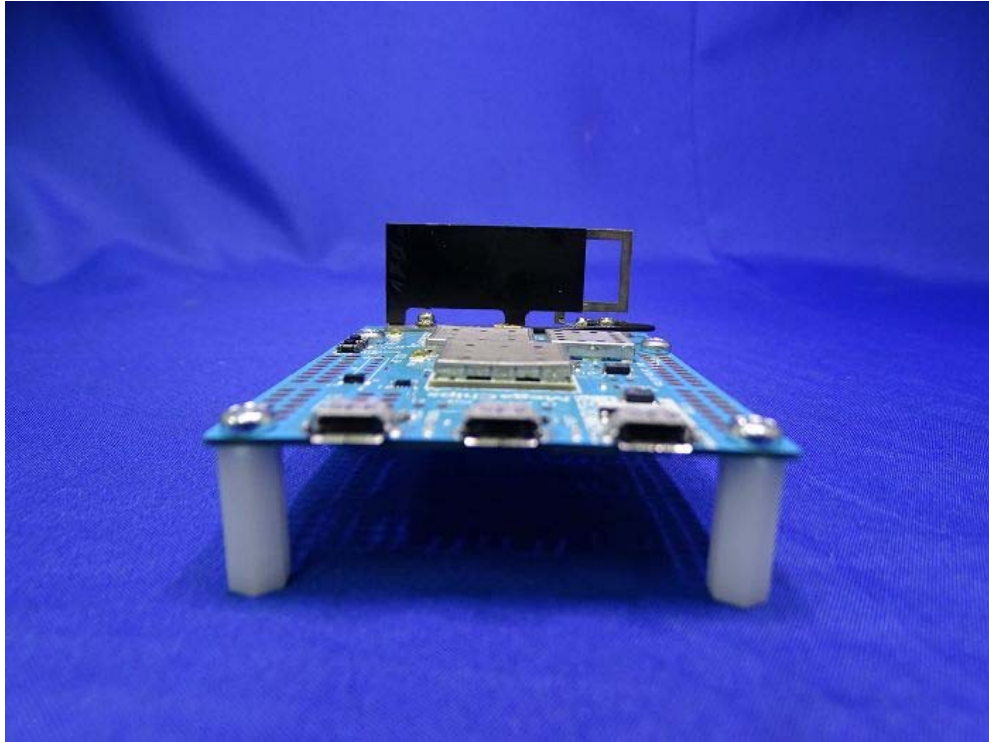
(3) EUT Photo
