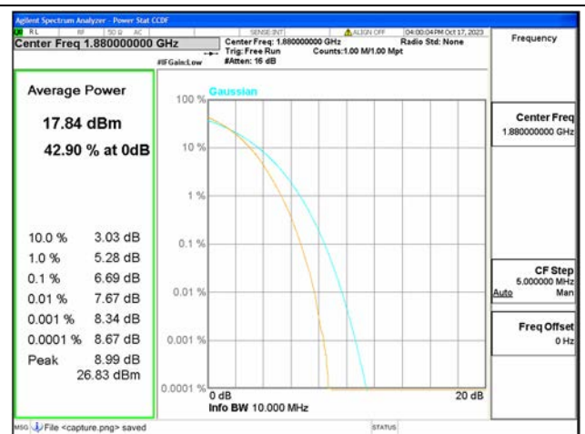
B2 / 10MHz / Mid CH / 256QAM
