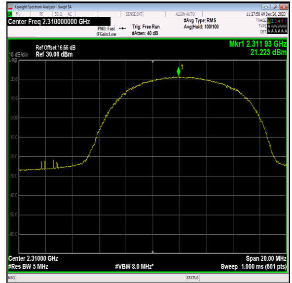
40(2305-2315)-10MHz-16QAM-38750-25RB#25-PASS
