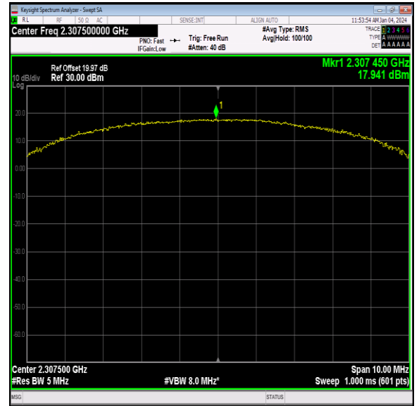
40(2305-2315)-5MHz-16QAM-38725-25RB#0-PASS
