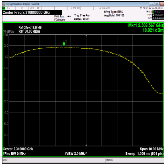
40(2305-2315)-5MHz-QPSK-38750-12RB#11-PASS
