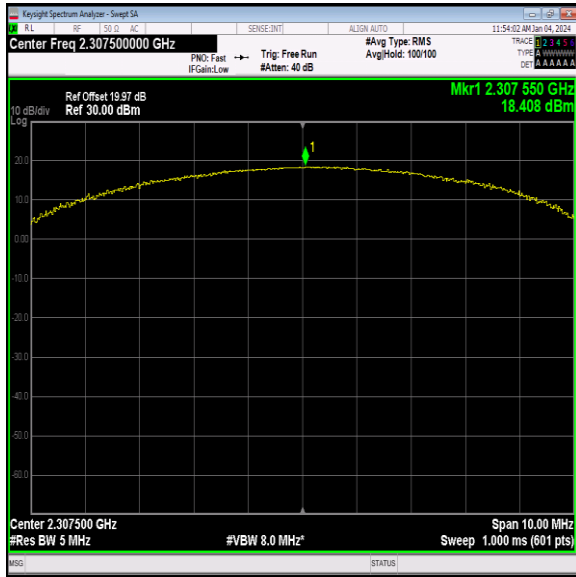
40(2305-2315)-5MHz-64QAM-38725-25RB#0-PASS
