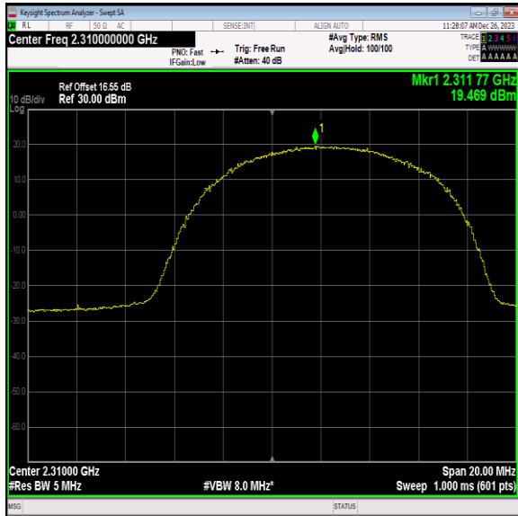
40(2305-2315)-10MHz-64QAM-38750-25RB#25-PASS
