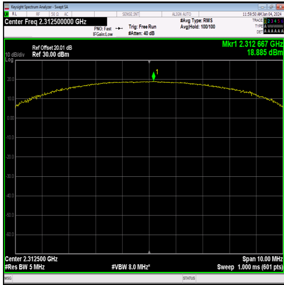
40(2305-2315)-5MHz-QPSK-38775-25RB#0-PASS
