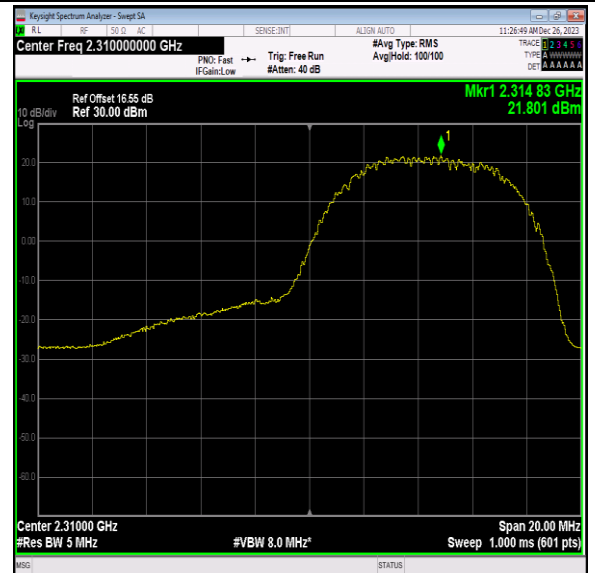
40(2305-2315)-10MHz-64QAM-38750-1RB#49-PASS
