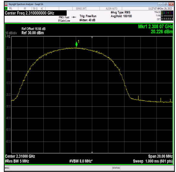
40(2305-2315)-10MHz-16QAM-38750-25RB#0-PASS
