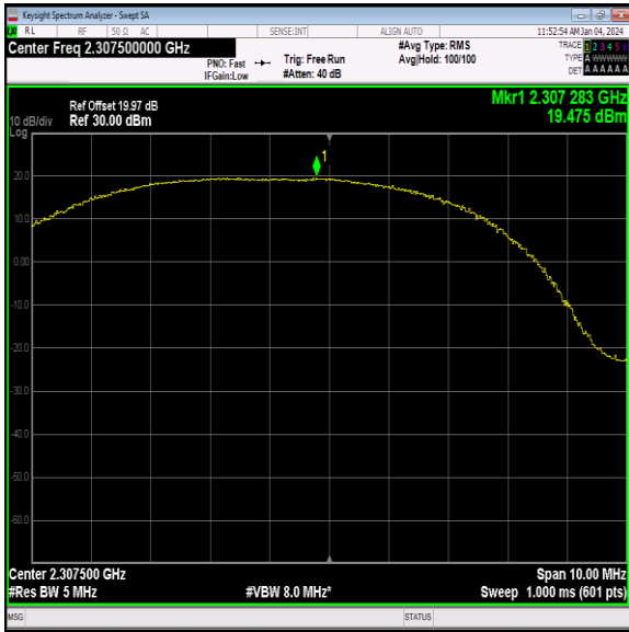
40(2305-2315)-5MHz-QPSK-38725-12RB#6-PASS
