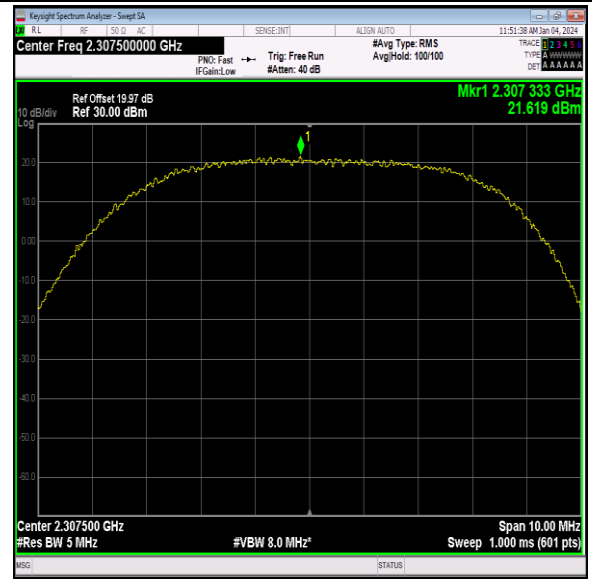
40(2305-2315)-5MHz-QPSK-38725-1RB#12-PASS
