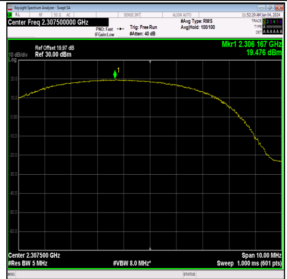
40(2305-2315)-5MHz-QPSK-38725-12RB#0-PASS
