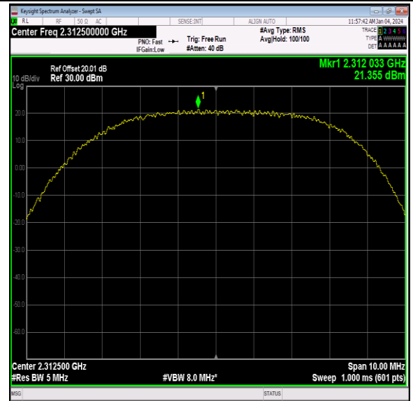
40(2305-2315)-5MHz-QPSK-38775-1RB#12-PASS
