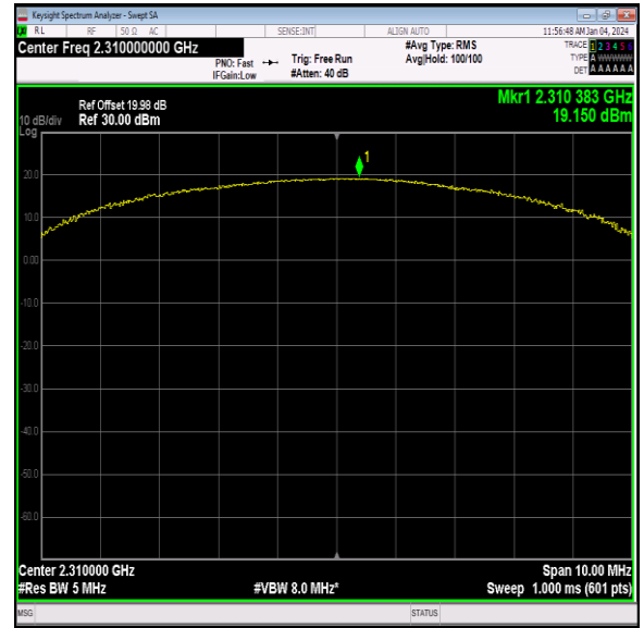
40(2305-2315)-5MHz-QPSK-38750-25RB#0-PASS
