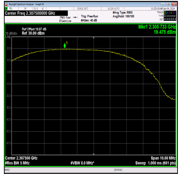
40(2305-2315)-5MHz-QPSK-38725-12RB#11-PASS
