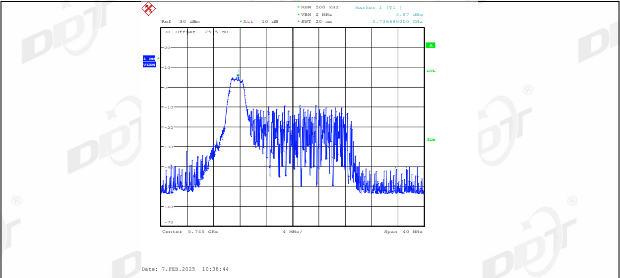
11AX20MIMO_Ant2_5745_26Tone_RU4
