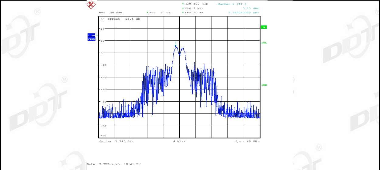
11AX20MIMO_Ant2_5745_26Tone_RU8
