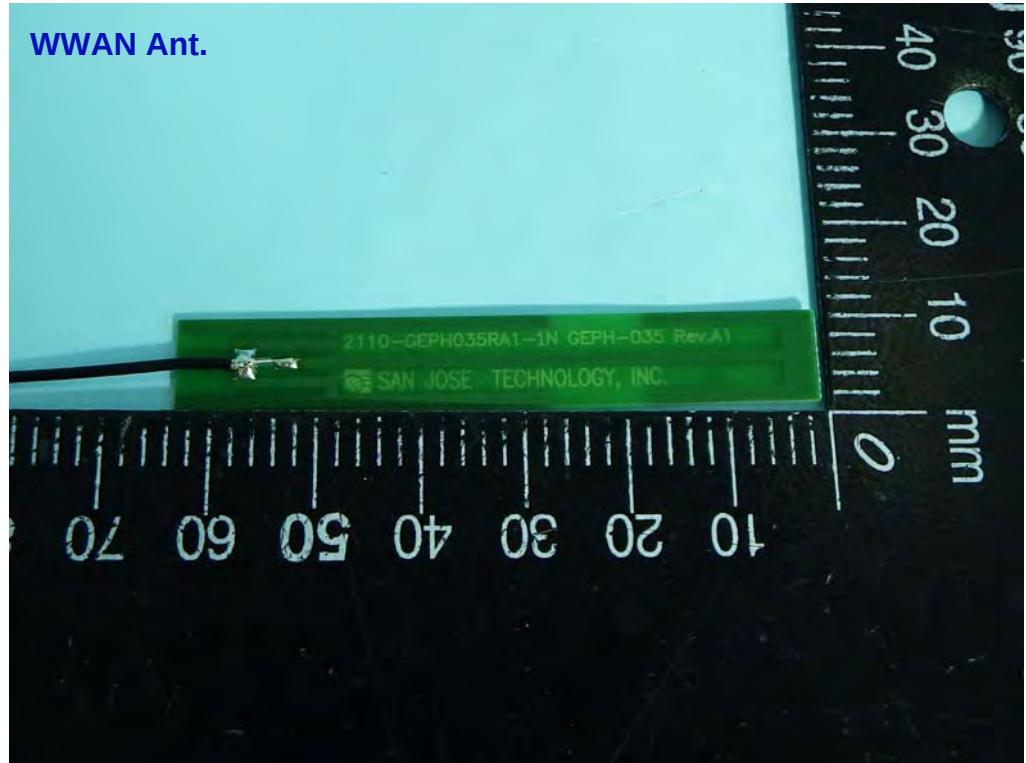
WWAN Ant.
