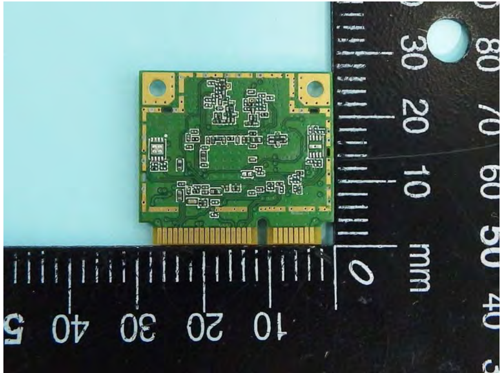
WWAN Module
