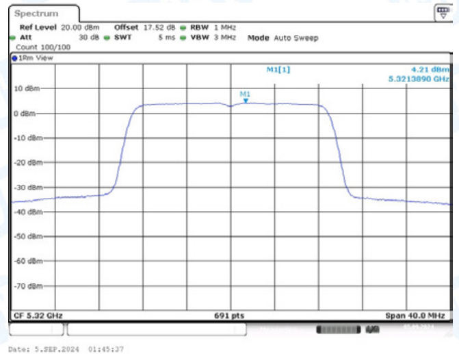
11AC20-CDD-Ant2-5320-PASS
