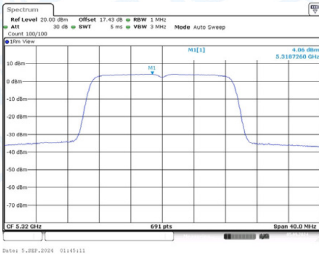
11AC20-CDD-Ant1-5320-PASS
