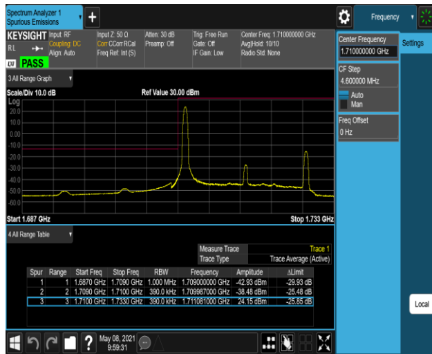
Band4-20MHz-QPSK-20050-100RB#0
