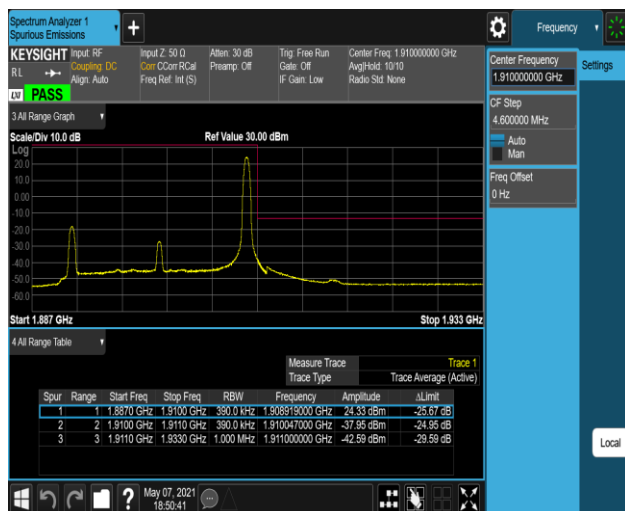
Band2-20MHz-16QAM-19100-1RB#99
