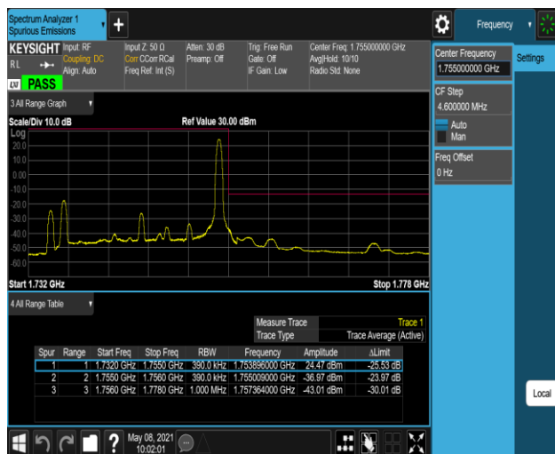
Band4-20MHz-QPSK-20300-1RB#99
