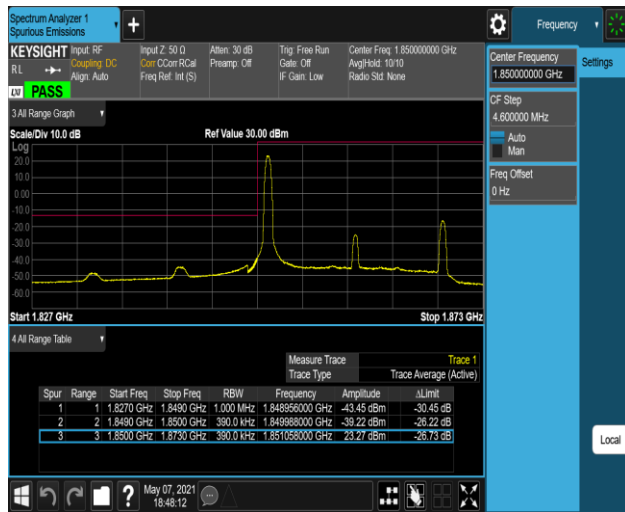
Band2-20MHz-16QAM-18700-100RB#0
