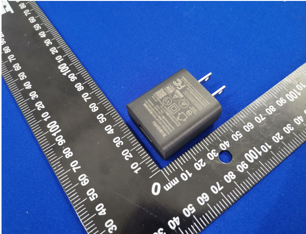
10) EUT Photo
