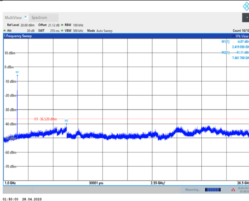
11G_Ant1_2417_0~Reference
