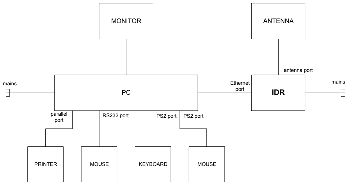
EUT test configuration
