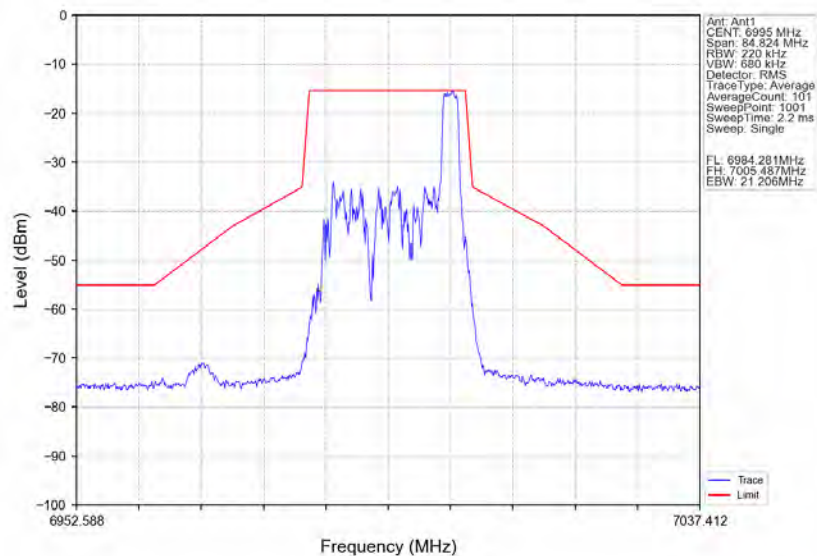
802.11ax(HE20)_MCH_6995MHz_RU26_Right_Ant1_NTNV
