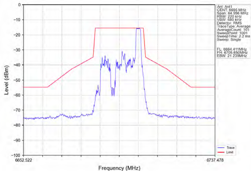
802.11ax(HE20)_MCH_6695MHz_RU26_Right_Ant1_NTNV
