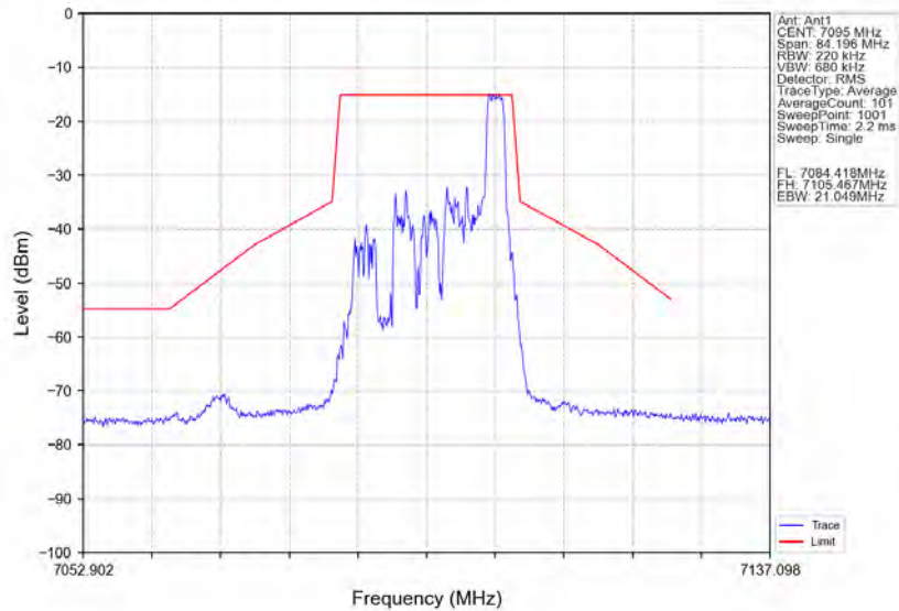
802.11ax(HE20) HCH_7095MHz_RU26_Right_Ant1_NTNV
