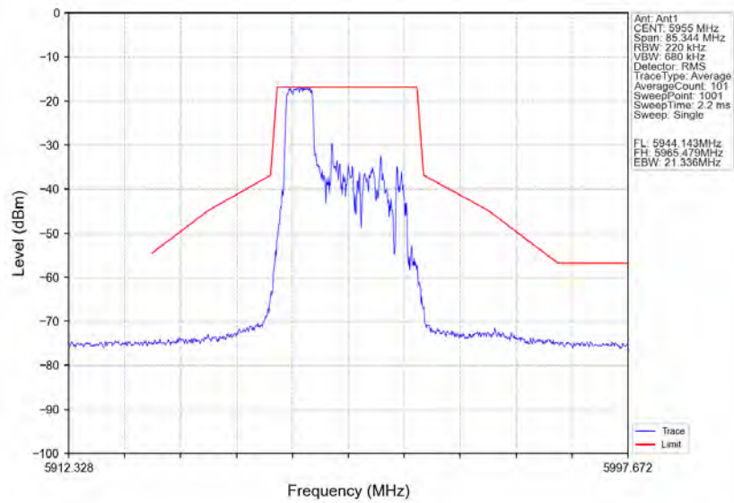
802.11ax(HE20)_LCH_5955MHz_RU52_Right_Ant1_NTNV
