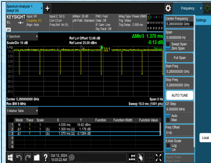
NTNV-11N20MIMO-Ant1-5280
