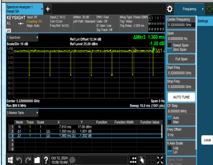
NTNV-11N20MIMO-Ant1-5320
