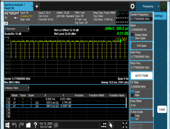
NTNV-11AC80SISO-Ant2-5775
