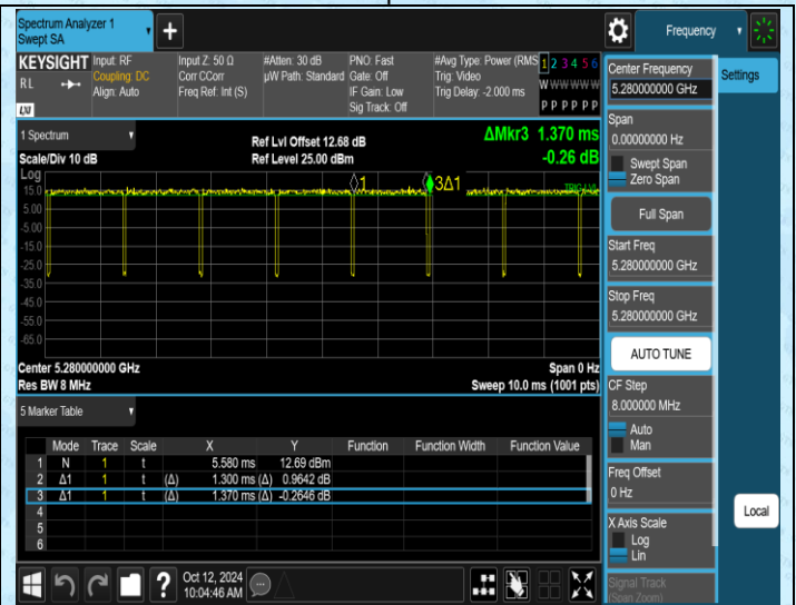
NTNV-11N20MIMO-Ant2-5280
