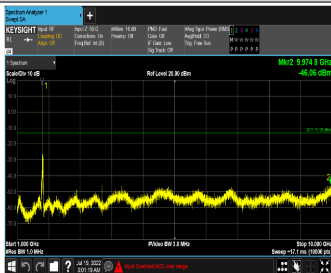
Band66-20MHz-QPSK-132072-1RB#0-Range5:1000~10000MHz
