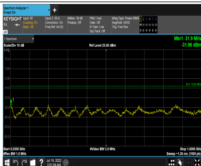
Band66-20MHz-QPSK-132072-1RB#0-Range1:30~1000MHz
