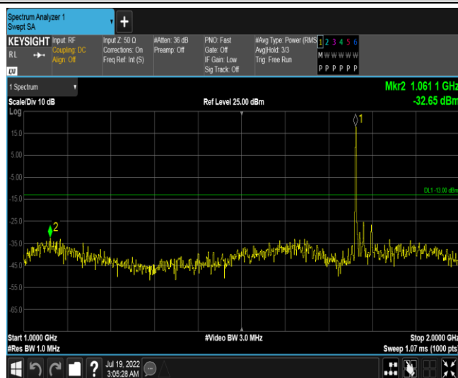
Band66-20MHz-QPSK-132572-1RB#0-Range2:1000~2000MHz
