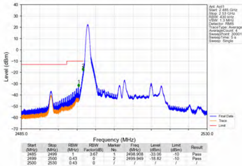
Band7_20MHz_QPSK_LCH_2510MHz_RB_1_0_NTNV
