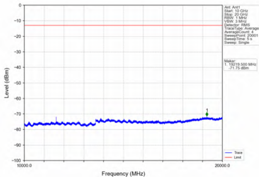
Band25 20MHz QPSK LCH 1860MHz RB 100 0 NTNV
