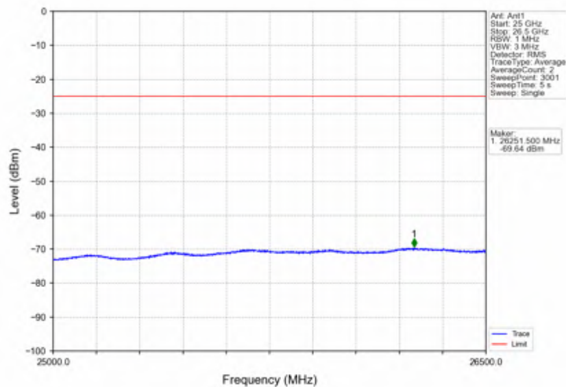
Band7_20MHz_16QAM_LCH_2510MHz_RB_100_0_NTNV
