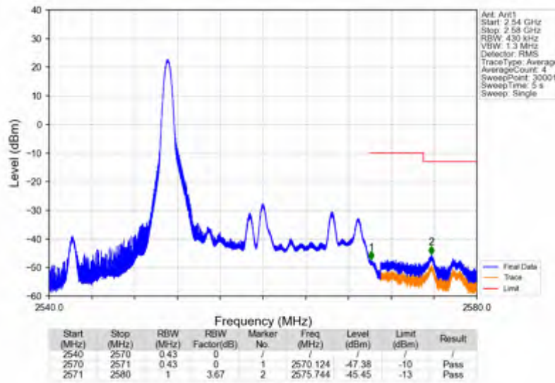
Band7_20MHz_64QAM_HCH_2560MHz_RB_100_0_NTNV
