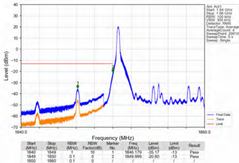
Band25_10MHz_QPSK_LCH_1855MHz_RB_1_0_NTNV
