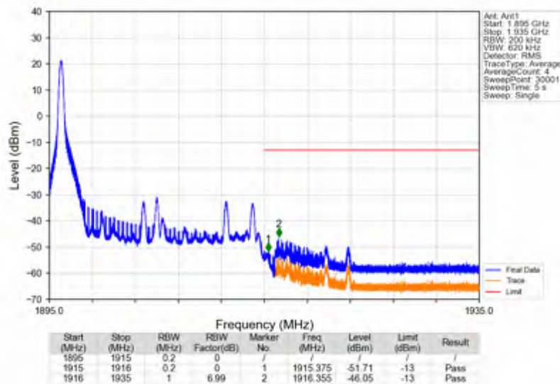
Band25_20MHz_QPSK_HCH_1905MHz_RB_100_0_NTNV
