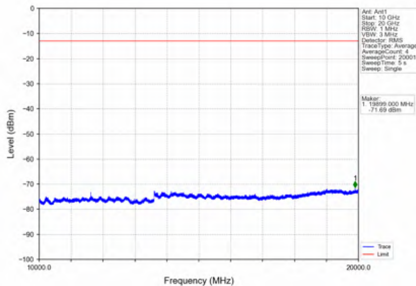
Band25 20MHz 16QAM HCH 1905MHz RB 1 0 NTNV
