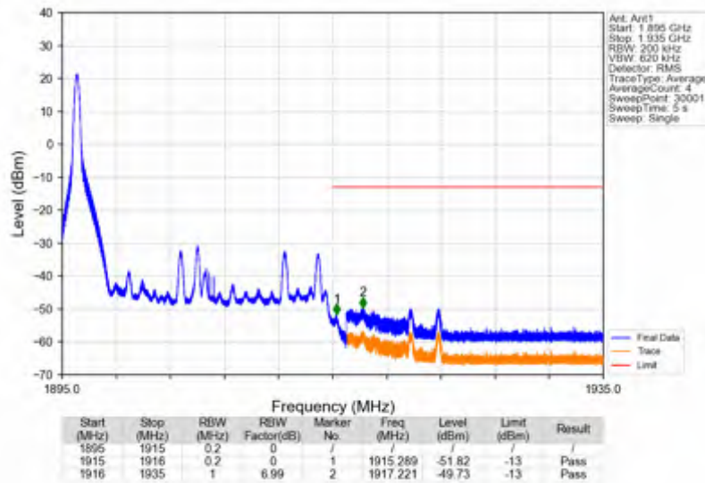
Band25_20MHz_QPSK_HCH_1905MHz_RB_1_99_NTNV
