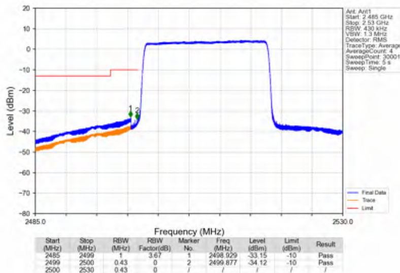
Band7_20MHz_256QAM_LCH_2510MHz_RB_100_0_NTNV
