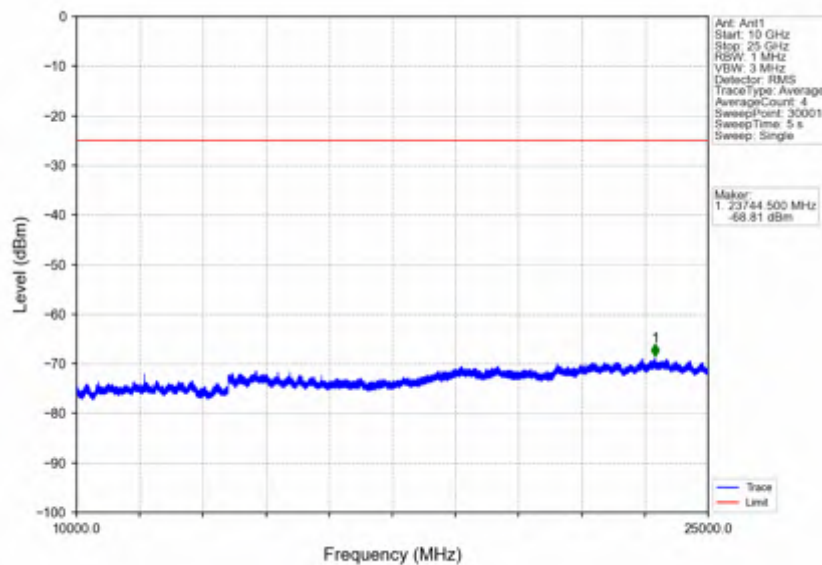
Band7_20MHz_64QAM_HCH_2560MHz_RB_1_0_NTNV
