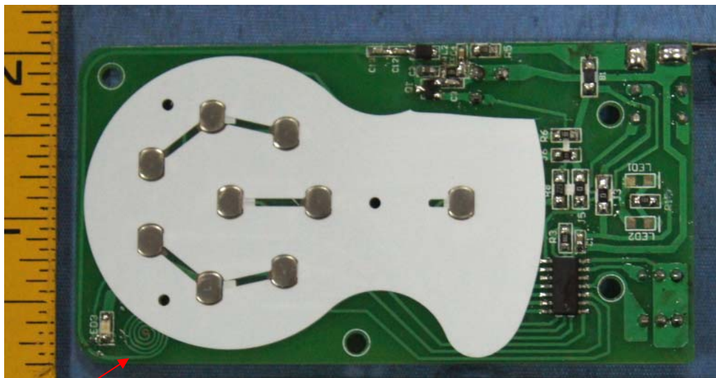
Antenna
