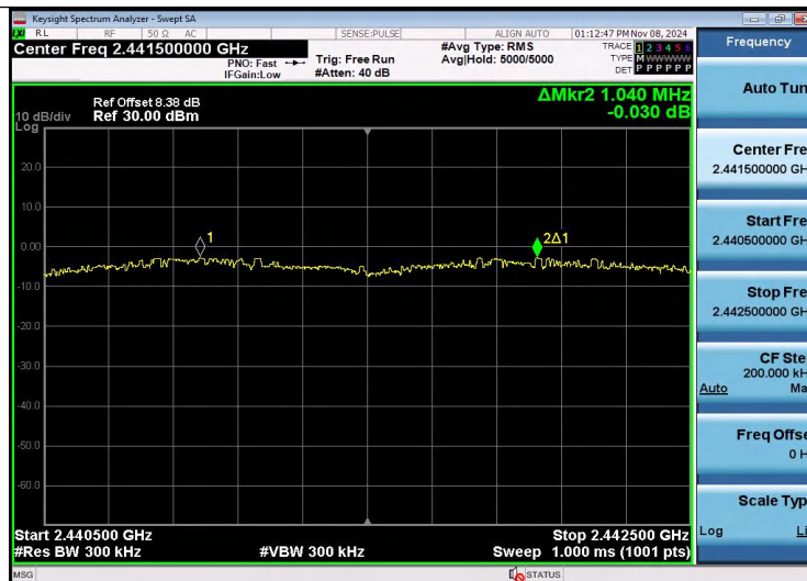
8DPSK
