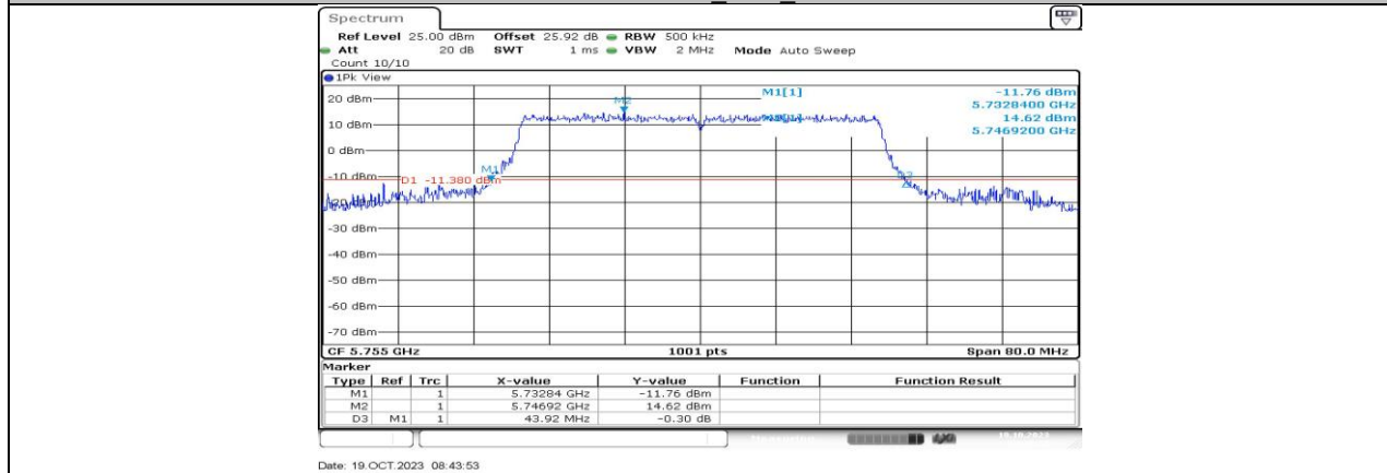
11AX40MIMO_Ant2_5755
