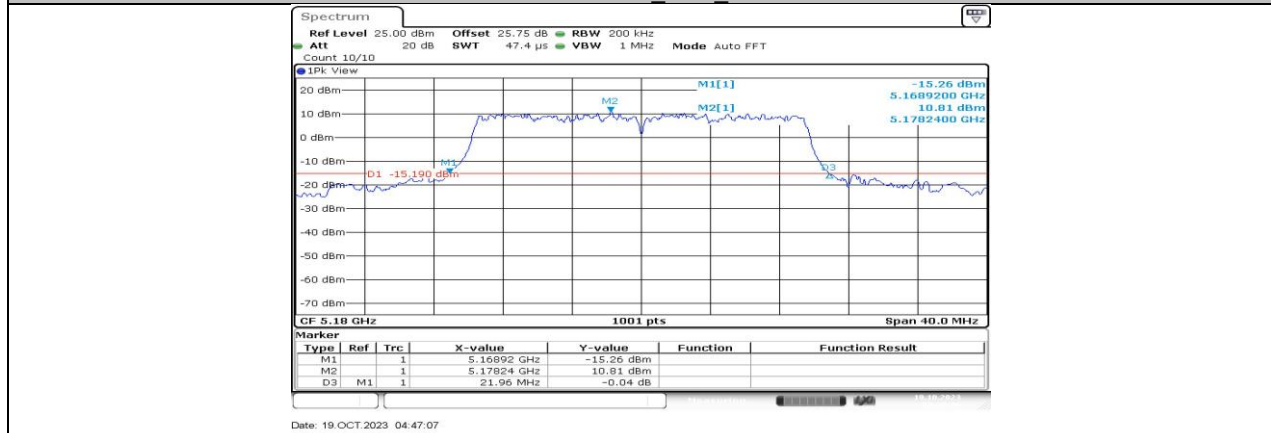
11AX20MIMO_Ant4_5180
