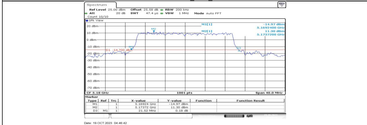
11AX20MIMO_Ant2_5180
