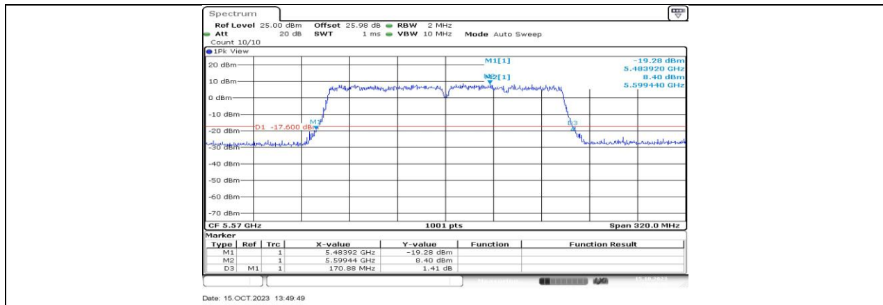
11AC160MIMO_Ant4_5570
