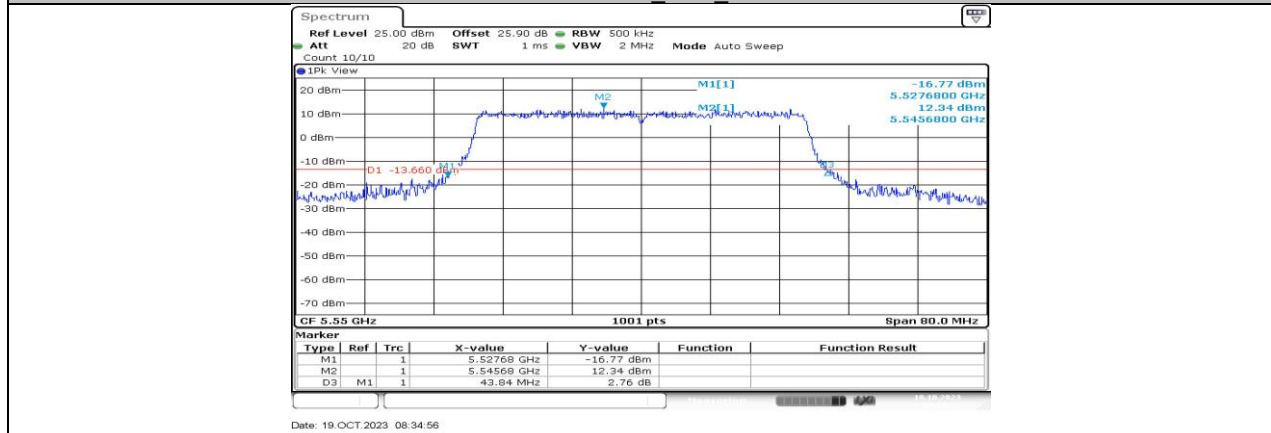
11AX40MIMO_Ant2_5550
