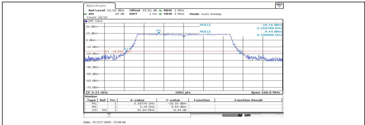
11AC80MIMO_Ant4_5210
