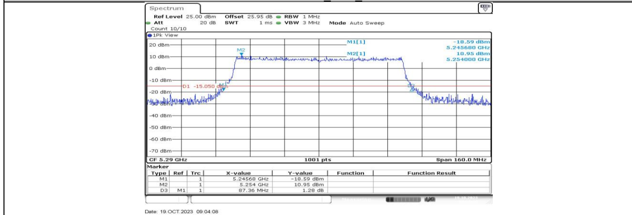
11AX80MIMO_Ant4_5290
