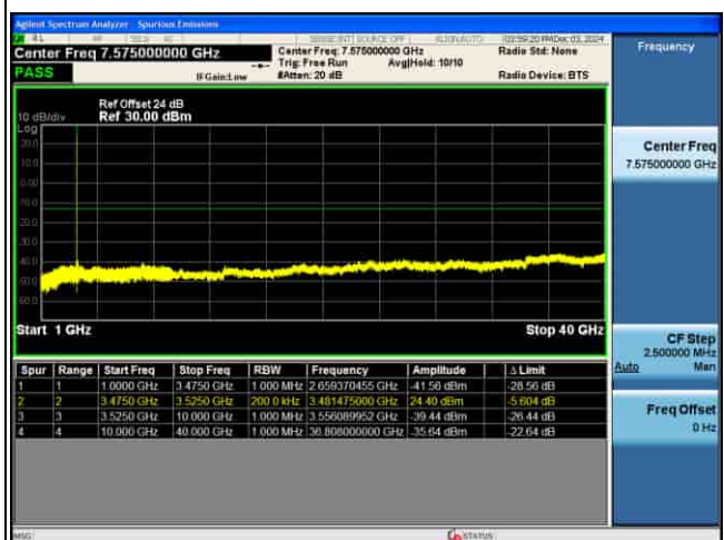
CSE_5G_n77(K)_30KHz_QPSK_40M CH633334_1RB@1_
