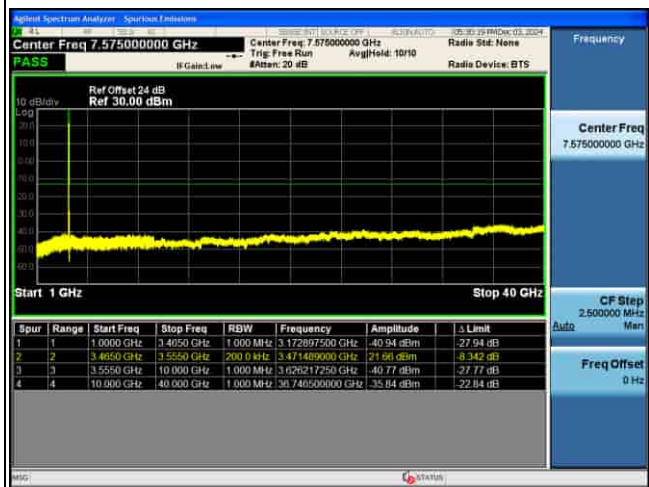
CSE_5G_n77(K)_30KHz_QPSK_90M CH633000_1RB@1_
