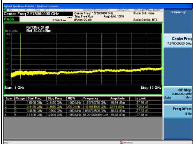
CSE_5G_n77(K)_30KHz_QPSK_30M CH633334_1RB@1_
