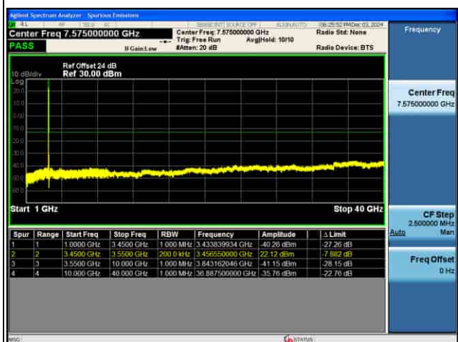
CSE_5G_n77(K)_30KHz_QPSK_90M CH633334_1RB@1_
