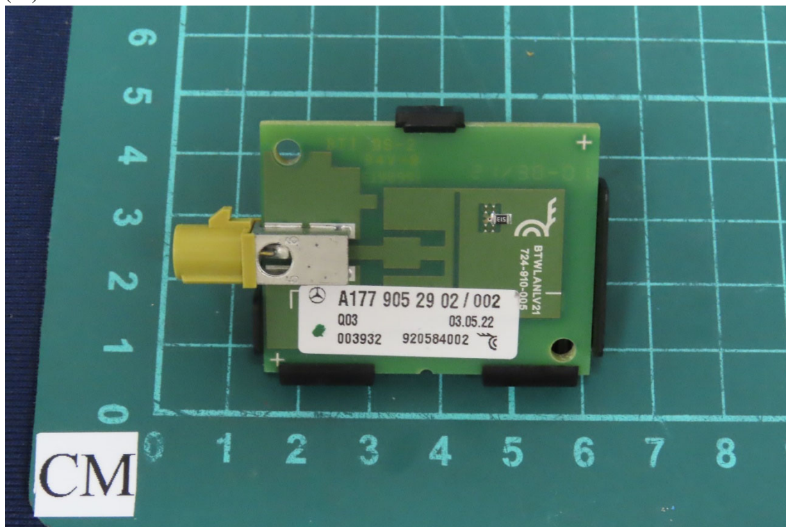
(10) EUT Photo
