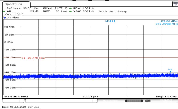
11N20MIMO_Ant4_2417_30-1000
