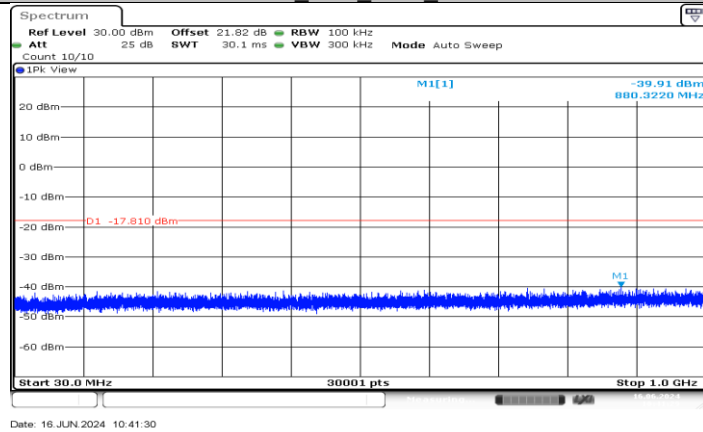
11AX20MIMO_Ant4_2457_30~1000
