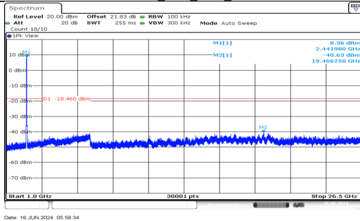
11N20MIMO_Ant3_2437_1000-26500
