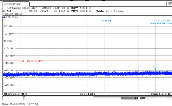
11N40MIMO_Ant4_2447_30-1000
