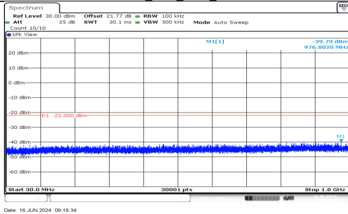
11AX20MIMO_Ant4_2412_30~1000
