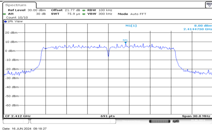
11AX20MIMO_Ant4_2412_0~Reference
