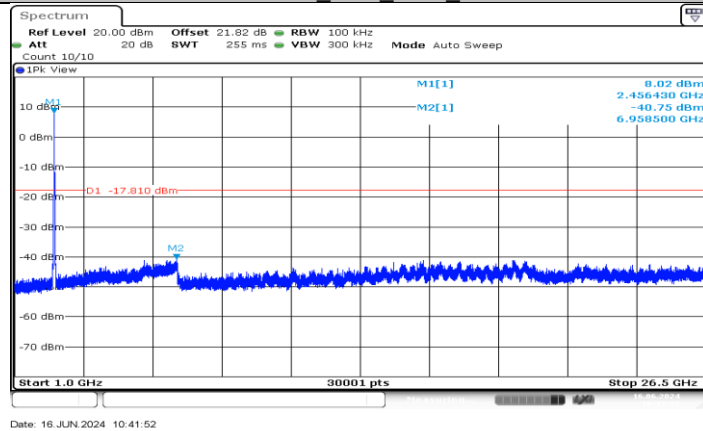
11AX20MIMO_Ant4_2457_1000~26500
