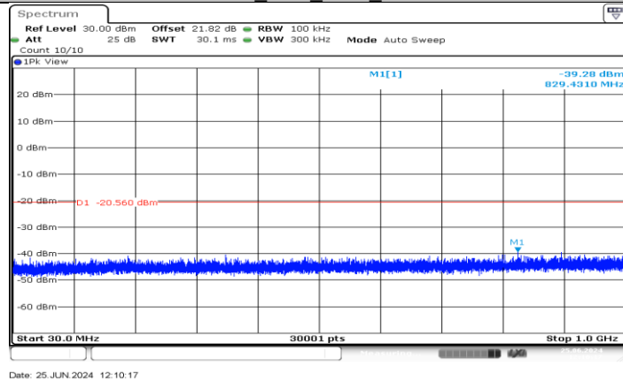
11N20MIMO_Ant4_2462_30-1000
