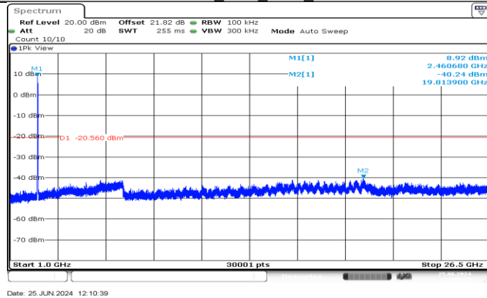
11N20MIMO_Ant4_2462_1000-26500
