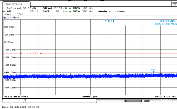
11B-CDD_Ant4_2462_30-1000
