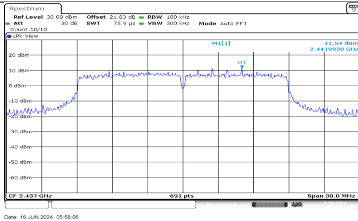
11N20MIMO_Ant3_2437_0-Reference
