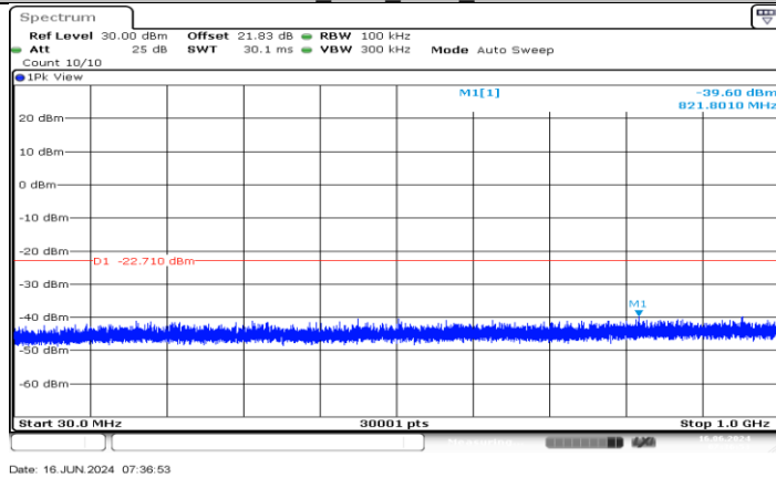
11N40MIMO_Ant3_2437_30-1000
