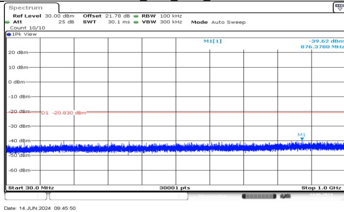
11N20MIMO_Ant3_2412_30-1000
