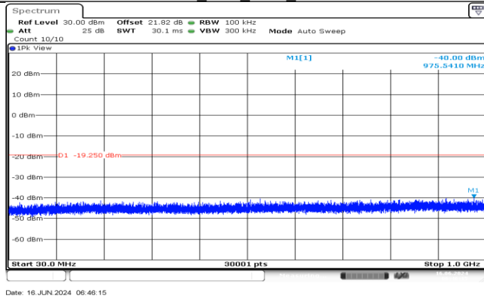
11N20MIMO_Ant4_2457_30-1000
