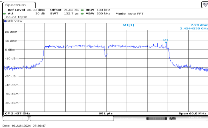
11N40MIMO_Ant3_2437_0-Reference
