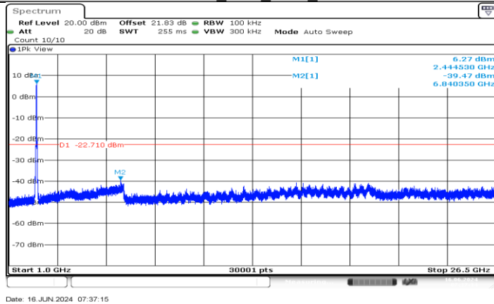
11N40MIMO_Ant3_2437_1000-26500
