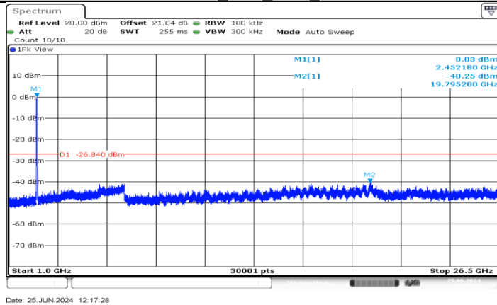
11N40MIMO_Ant4_2447_1000-26500
