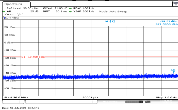
11N20MIMO_Ant3_2437_30-1000
