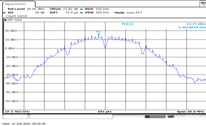
11B-CDD_Ant4_2462_0-Reference
