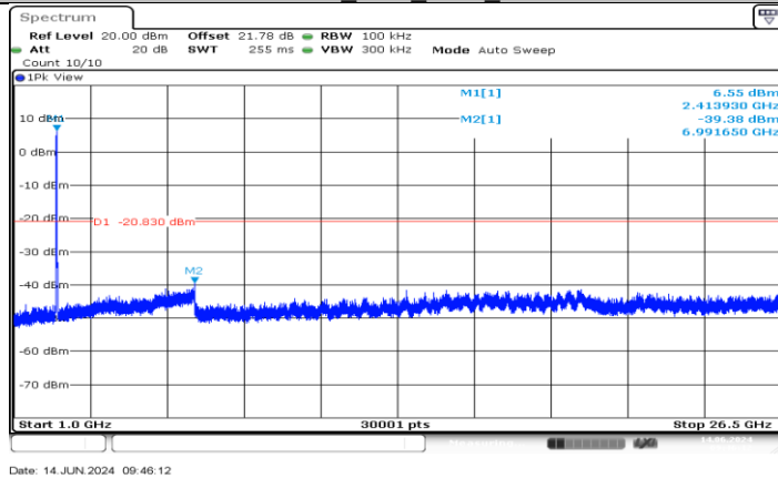
11N20MIMO_Ant3_2412_1000-26500
