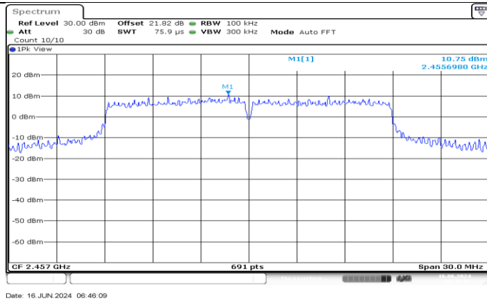
11N20MIMO_Ant4_2457_0-Reference
