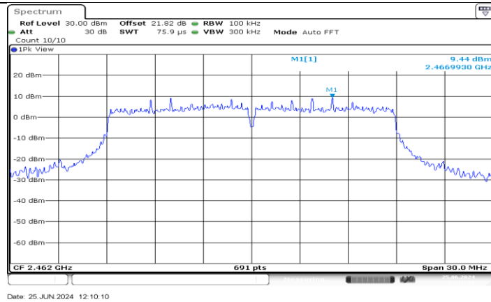
11N20MIMO_Ant4_2462_0-Reference
