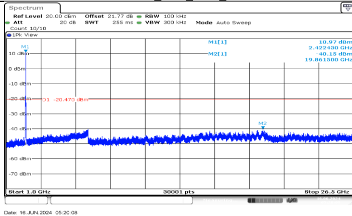
11N20MIMO_Ant4_2417_1000-26500
