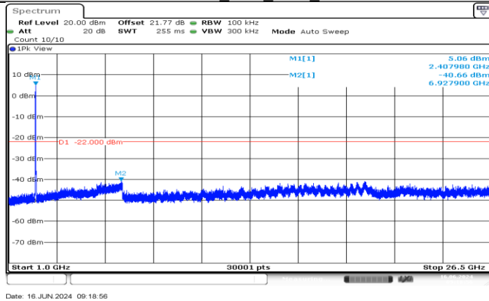
11AX20MIMO_Ant4_2412_1000~26500
