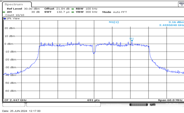
11N40MIMO_Ant4_2447_0-Reference
