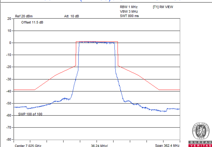
802.11be (EHT80) / Chain 1 : CH 215
