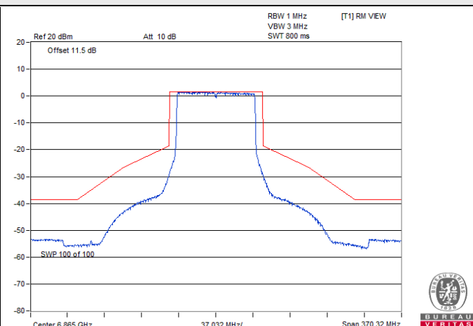
802.11be (EHT80) / Chain 1 : CH 183
