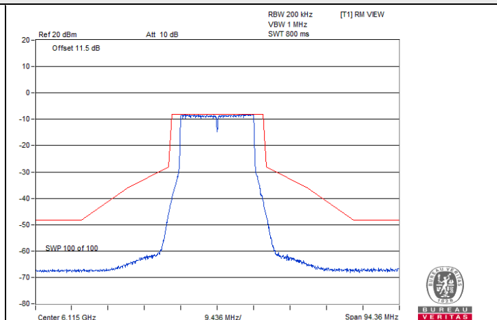
802.11be (EHT20) / Chain 1 : CH 33
