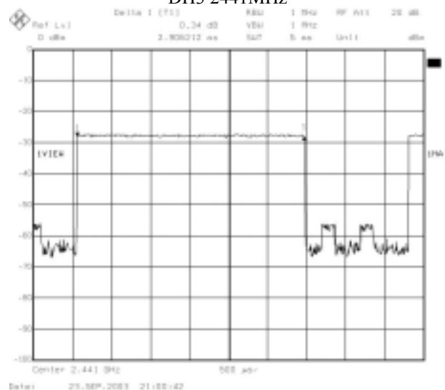
DH5 2441MHz
