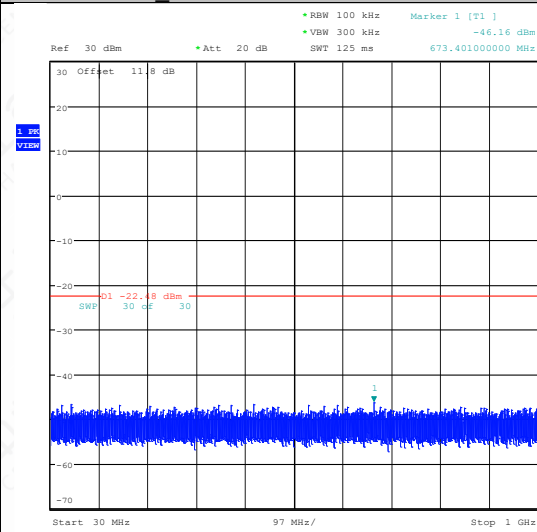
BLE_2M-Ant1-2440-30~1000-PASS
