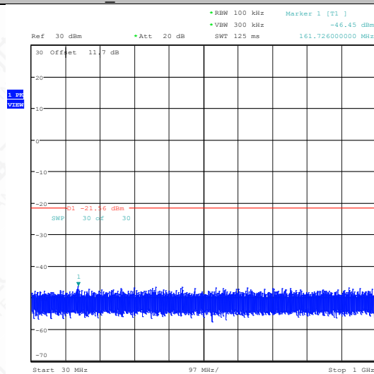
BLE_2M-Ant1-2402-30~1000-PASS
