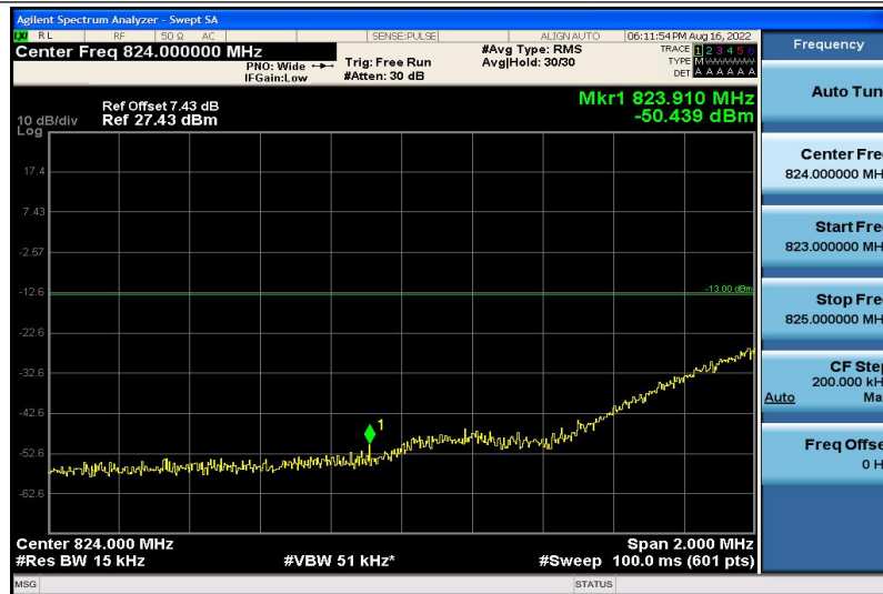
Band5-3MHz-QPSK-20415-1RB#5
