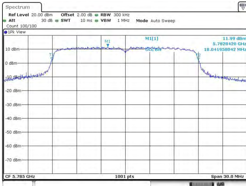
11N20MIMO_Ant1_5785
