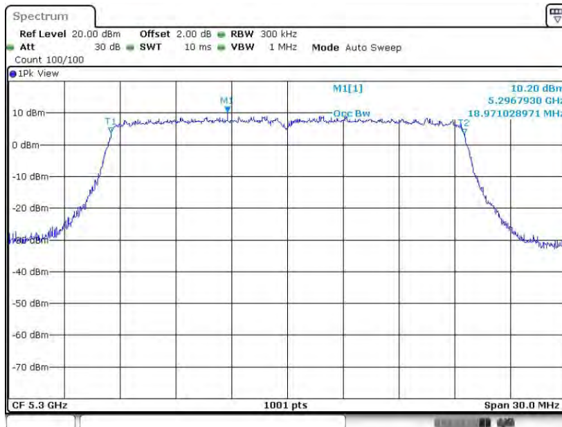
11AX20MIMO_Ant2_5300
