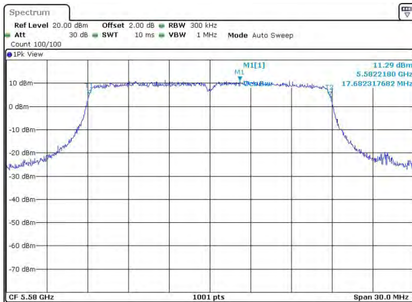
11N20MIMO_Ant2_5580
