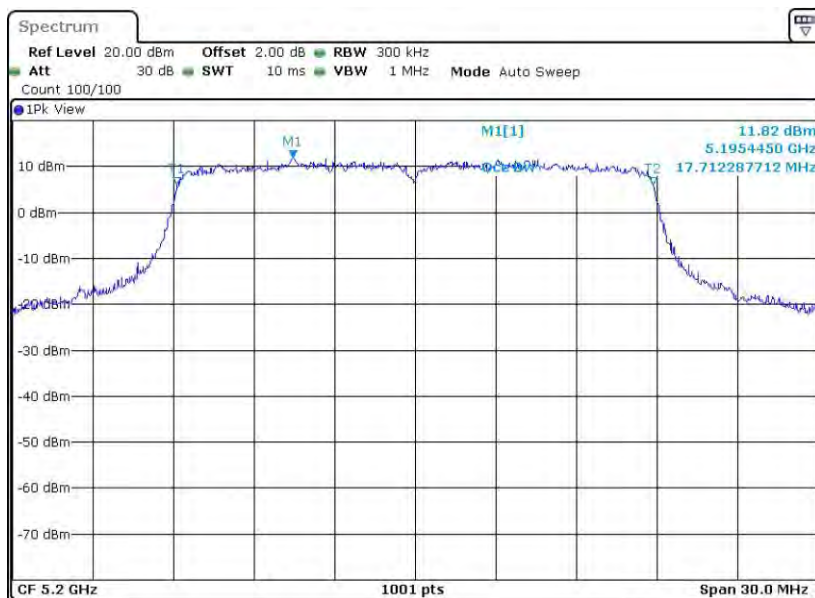
11AC20MIMO_Ant1_5200
