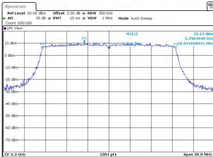
11AX20MIMO_Ant1_5300
