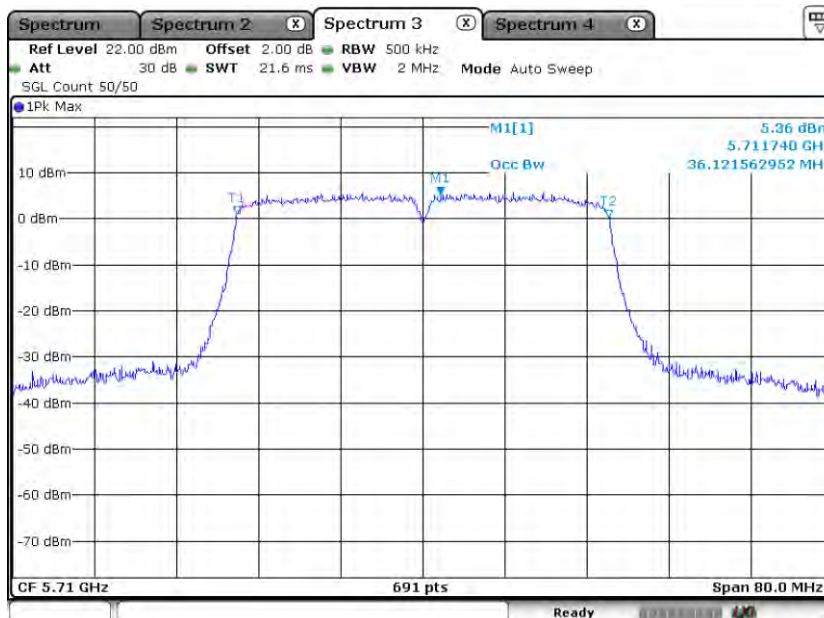
11N40MIMO_Ant1_5710
