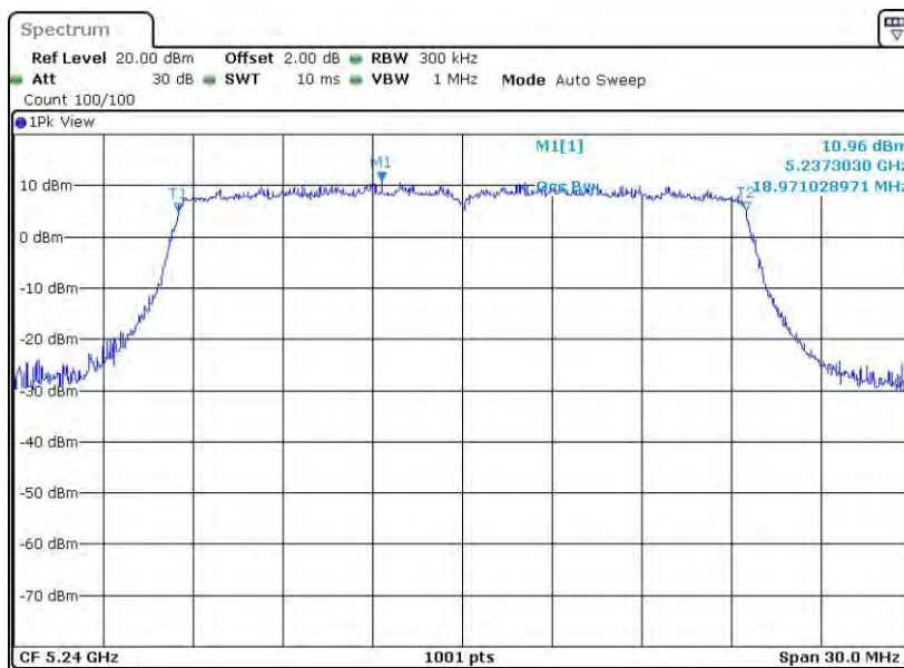
11AX20MIMO_Ant1_5240
