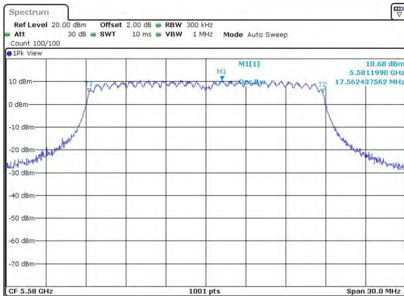
11AC20MIMO_Ant2_5580
