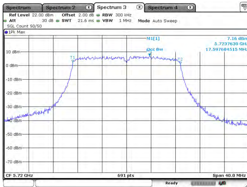
11N20MIMO_Ant2_5720
