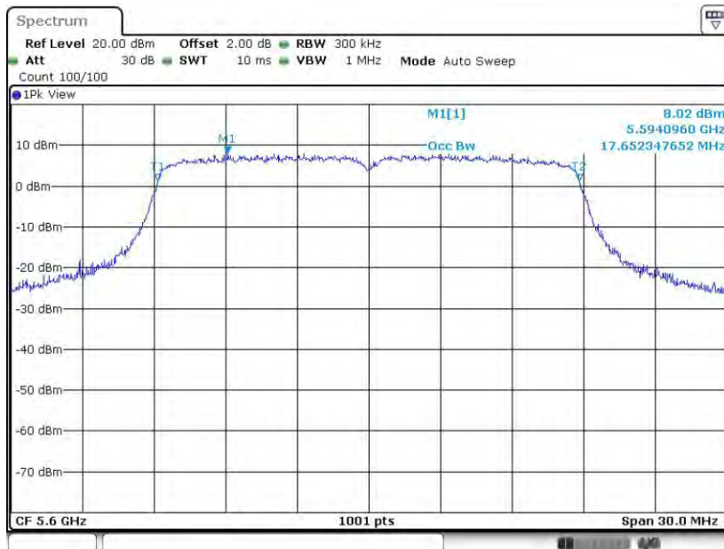
11N20MIMO_Ant1_5600
