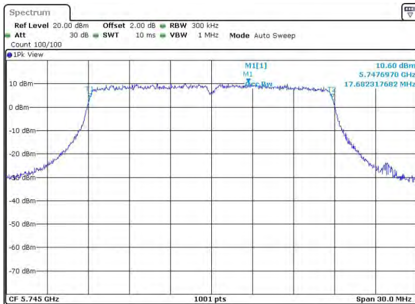
11N20MIMO_Ant2_5745
