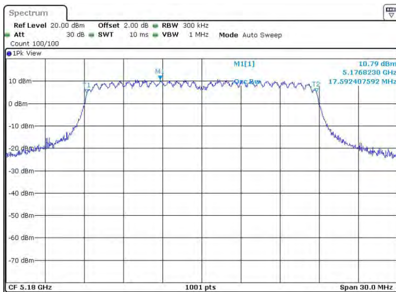
11AC20MIMO_Ant2_5180
