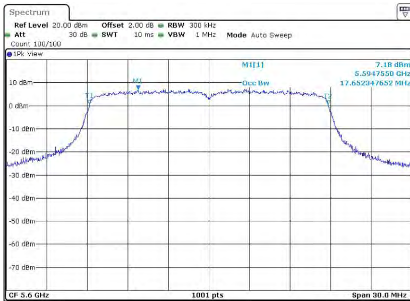
11AC20MIMO_Ant2_5600
