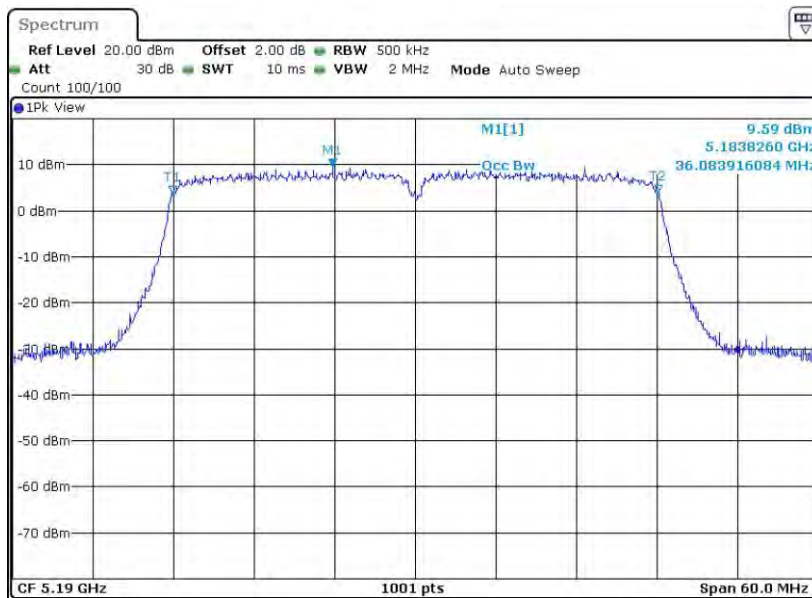
11N40MIMO_Ant2_5190
