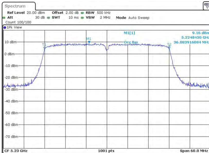
11N40MIMO_Ant1_5230
