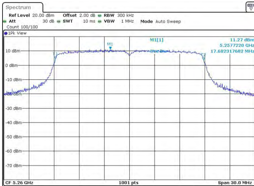
11N20MIMO_Ant1_5260
