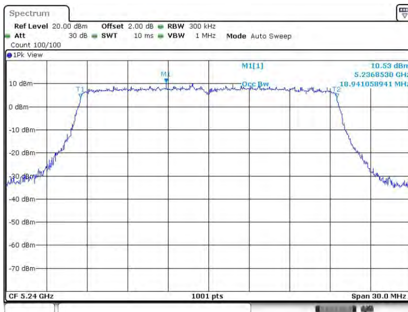
11AX20MIMO_Ant2_5240
