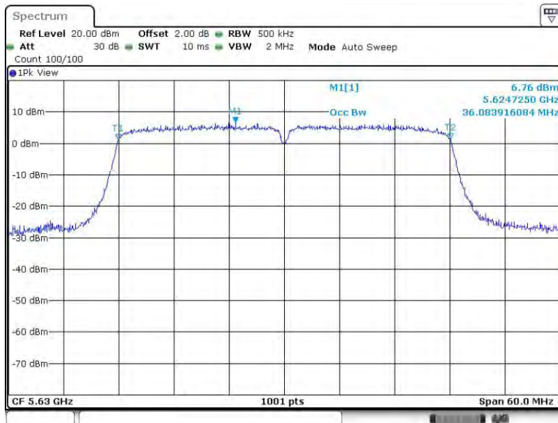
11N40MIMO_Ant1_5630
