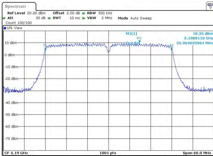
11AC40MIMO_Ant2_5190
