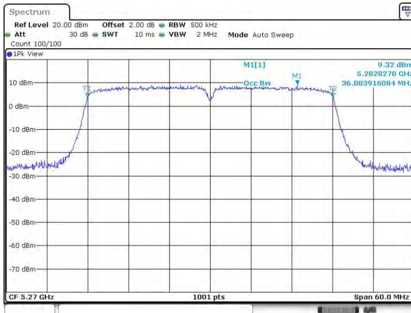
11AC40MIMO_Ant1_5270
