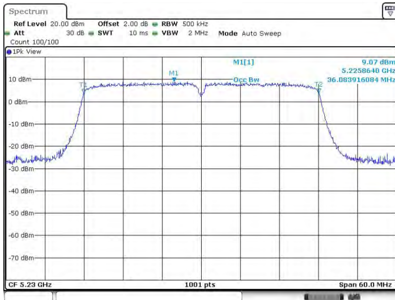
11AC40MIMO_Ant1_5230
