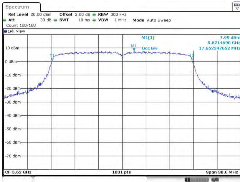
11AC20MIMO_Ant1_5620
