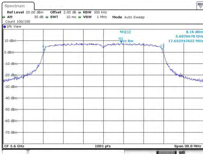
11AC20MIMO_Ant1_5600
