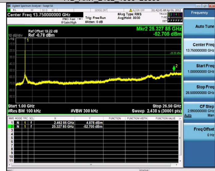
11B_Ant1_2462_1000~26500
