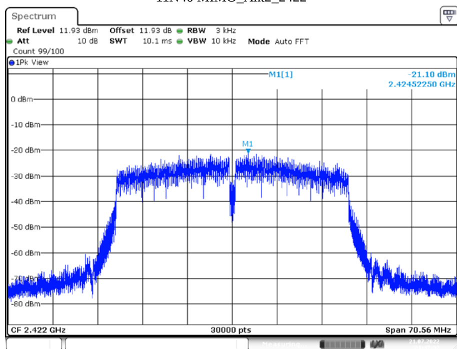
11N40 MIMO_Ant2_2422
