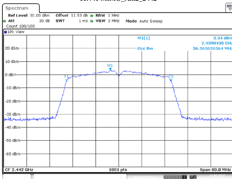
11N40 MIMO_Ant2_2442
