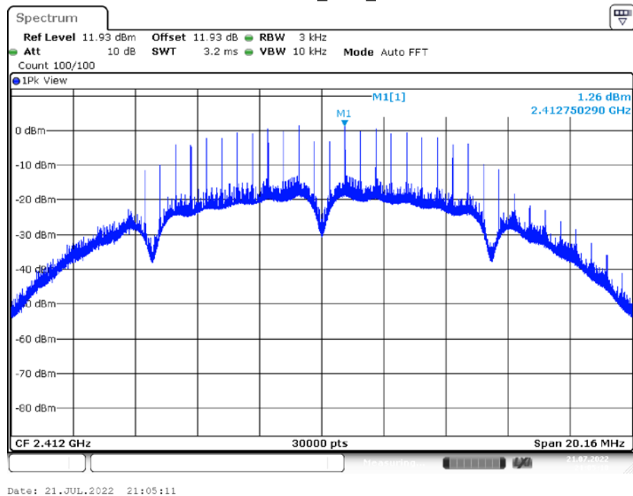
11B MIMO_Ant2_2412
