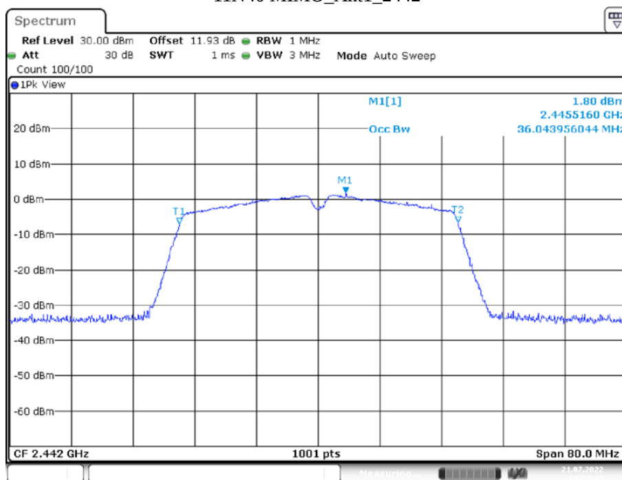
11N40 MIMO_Ant1_2442
