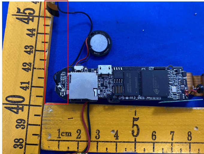
Antenna
