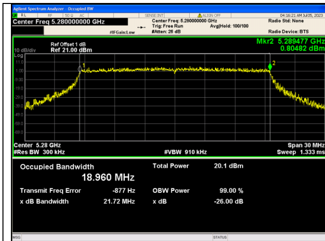
IEEE 802.11ax_Channel 56_20MHz_Antenna 0_RU&amp;Index 242RU61
