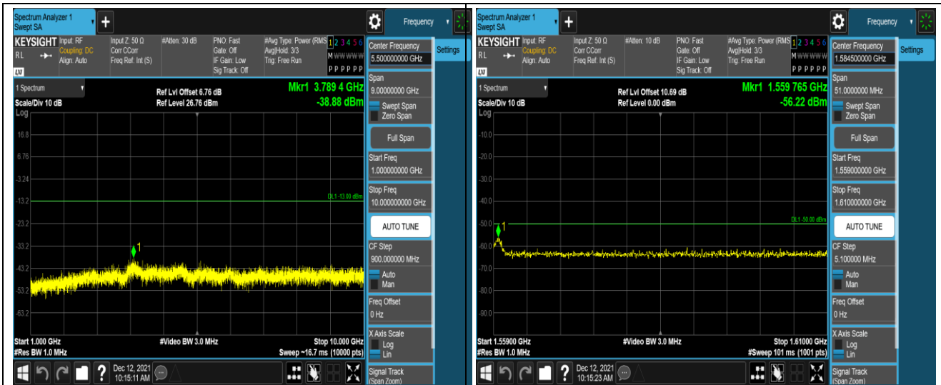
Band13-5MHz-QPSK-23230-1RB#0-Range2:1000~10000MHz
