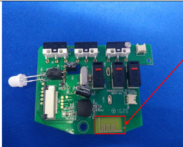
Antenna
