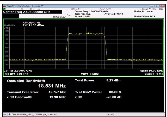
Figure 226: 64QAM 20MHz B.W.; 2506.0MHz, 30kHz Input
