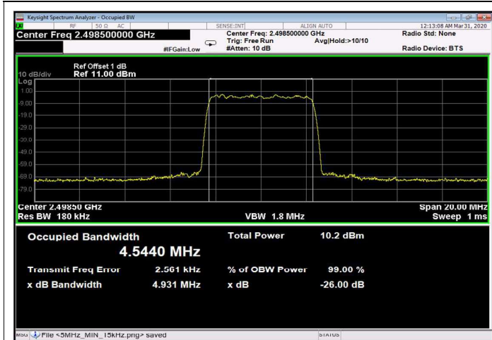
Figure 201: 64QAM 5MHz B.W.; 2498.5MHz, 15kHz Input
