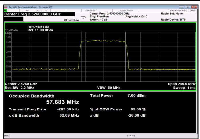
Figure 244: 64QAM 60MHz B.W.; 2526.0MHz, 60kHz Input
