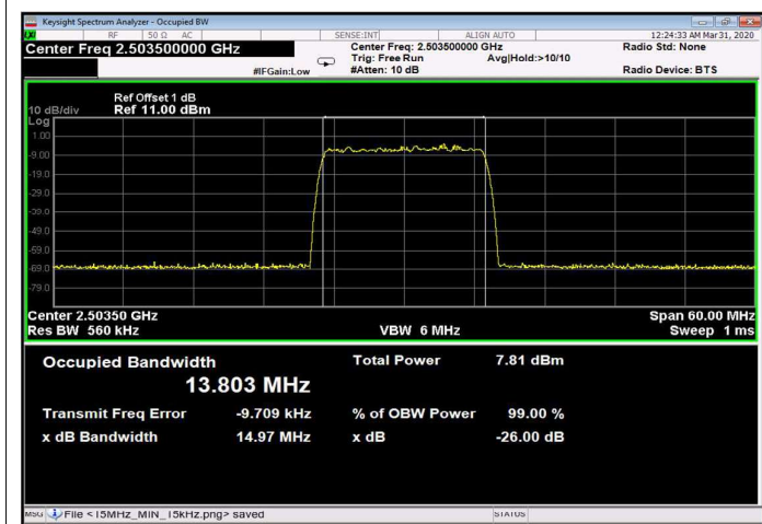
Figure 217: 64QAM 15MHz B.W.; 2503.5MHz, 30kHz Input
