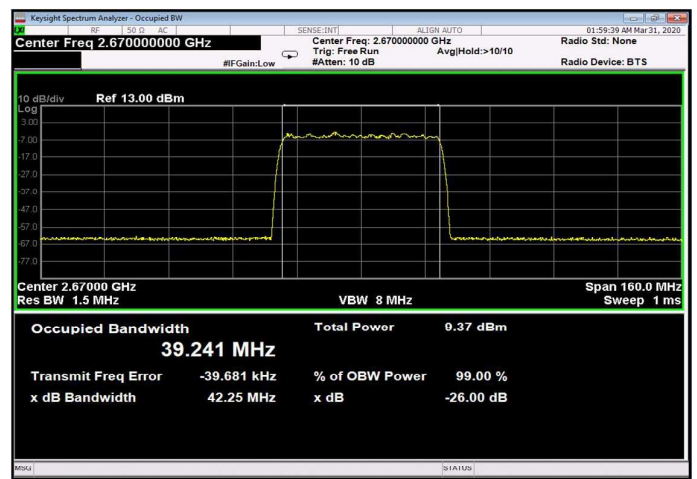
Figure 240: 64QAM 40MHz B.W.; 2670.0MHz, 15kHz Input
