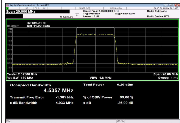
Figure 203: 64QAM 5MHz B.W.; 2593.0MHz, 15kHz Input
