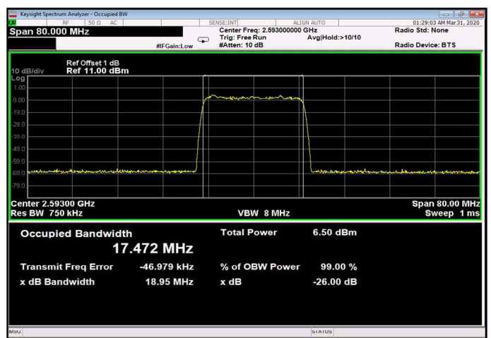
Figure 230: 64QAM 20MHz B.W.; 2593.0MHz, 60kHz Input
