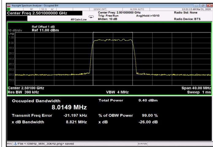
Figure 209: 64QAM 10MHz B.W.; 2501.0MHz, 60kHz Input
