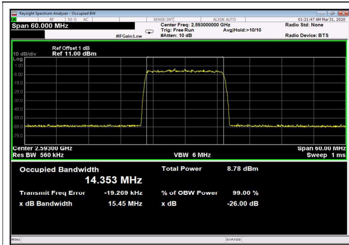
Figure 219: 64QAM 15MHz B.W.; 2593.0MHz, 15kHz Input
