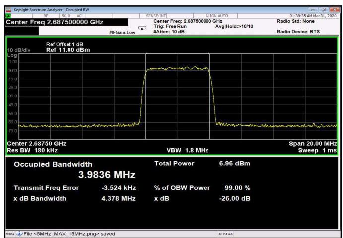
Figure 206: 64QAM 5MHz B.W.; 2687.5MHz, 30kHz Input
