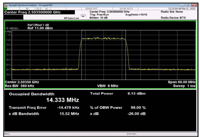
Figure 216: 64QAM 15MHz B.W.; 2503.5MHz, 15kHz Input
