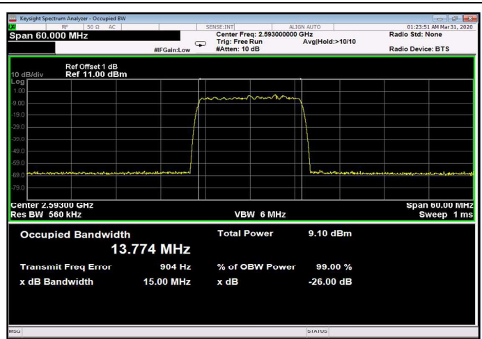
Figure 220: 64QAM 15MHz B.W.; 2593.0MHz, 30kHz Input
