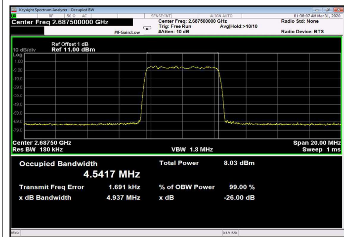
Figure 205: 64QAM 5MHz B.W.; 2687.5MHz, 15kHz Input
