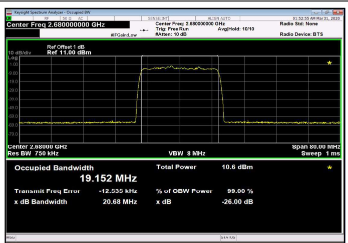
Figure 232: 64QAM 20MHz B.W.; 2680.0MHz, 30kHz Input
