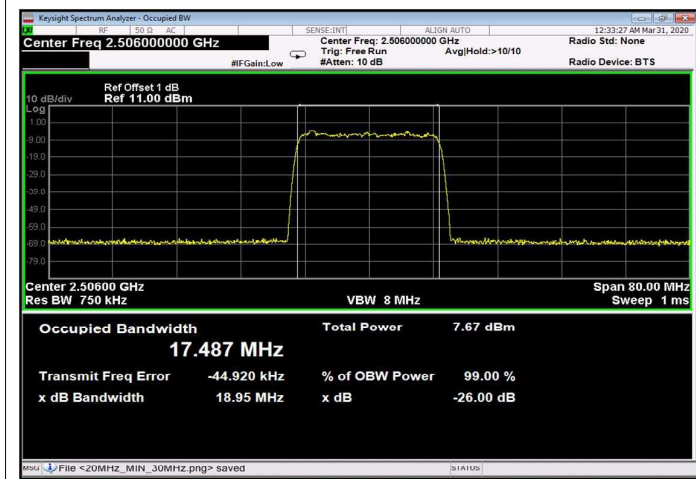
Figure 227: 64QAM 20MHz B.W.; 2506.0MHz, 60kHz Input
