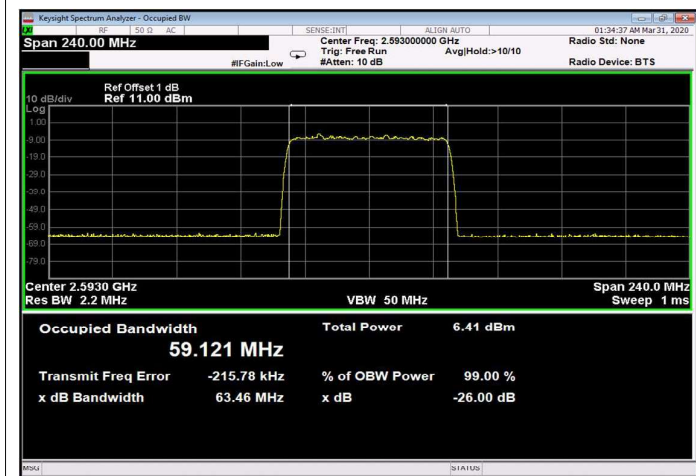
Figure 245: 64QAM 60MHz B.W.; 2593.0MHz, 30kHz Input
