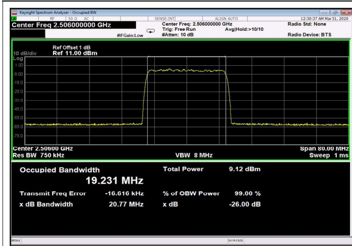
Figure 225: 64QAM 20MHz B.W.; 2506.0MHz, 15kHz Input
