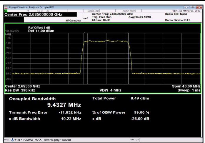
Figure 214: 64QAM 10MHz B.W.; 2685.0MHz, 30kHz Input
