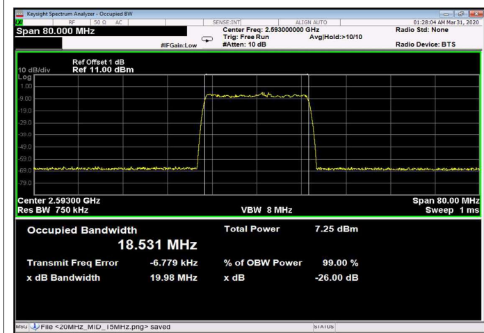
Figure 229: 64QAM 20MHz B.W.; 2593.0MHz, 30kHz Input
