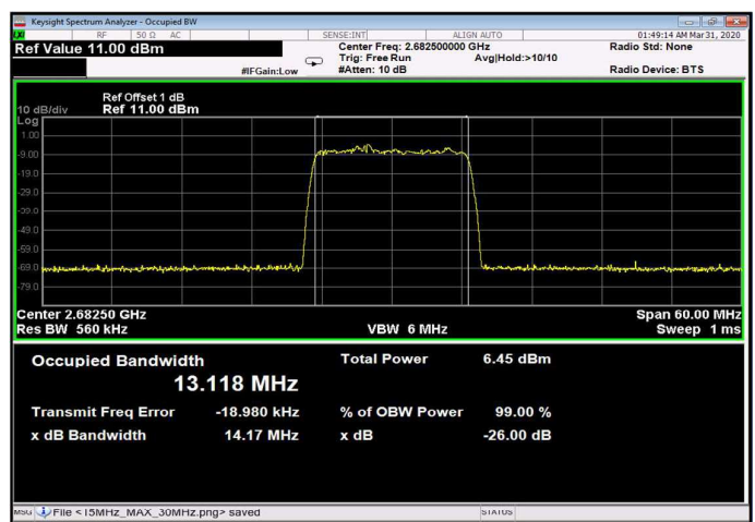
Figure 224: 64QAM 15MHz B.W.; 2682.5MHz, 60kHz Input
