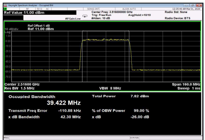
Figure 234: 64QAM 40MHz B.W.; 2516.0MHz, 15kHz Input
