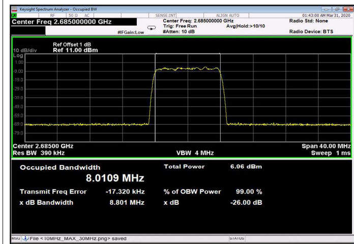
Figure 215: 64QAM 10MHz B.W.; 2685.0MHz, 60kHz Input
