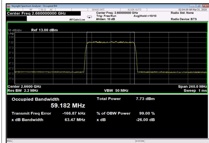
Figure 247: 64QAM 60MHz B.W.; 2660.0MHz, 30kHz Input
