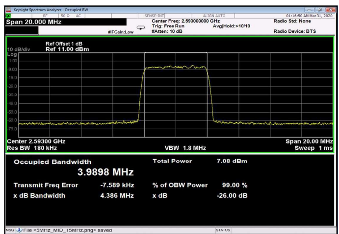
Figure 204: 64QAM 5MHz B.W.; 2593.0MHz, 30kHz Input
