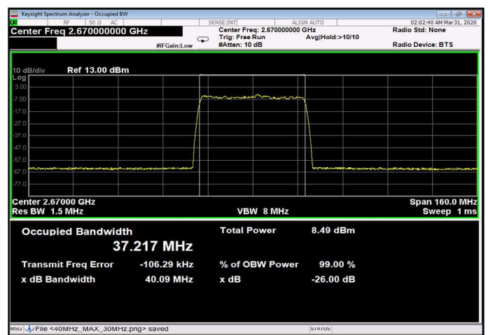
Figure 242: 64QAM 40MHz B.W.; 2670.0MHz, 60kHz Input
