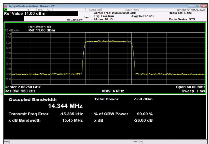
Figure 222: 64QAM 15MHz B.W.; 2682.5MHz, 15kHz Input
