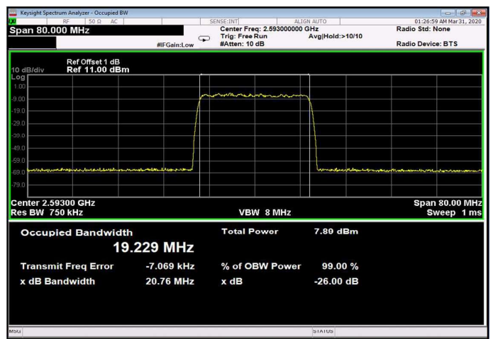
Figure 228: 64QAM 20MHz B.W.; 2593.0MHz, 15kHz Input
