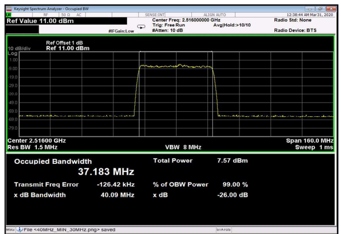
Figure 236: 64QAM 40MHz B.W.; 2516.0MHz, 60kHz Input
