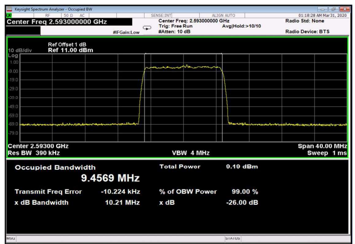
Figure 210: 64QAM 10MHz B.W.; 2593.0MHz, 15kHz Input
