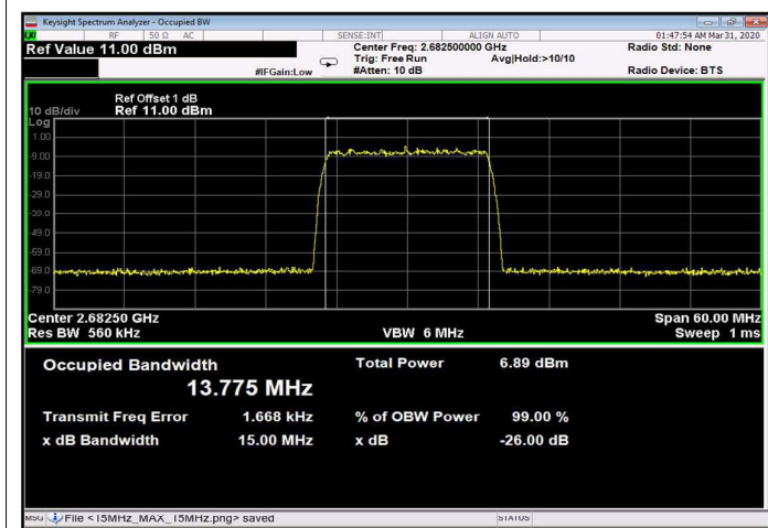
Figure 223: 64QAM 15MHz B.W.; 2682.5MHz, 30kHz Input
