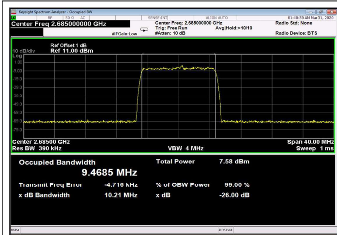
Figure 213: 64QAM 10MHz B.W.; 2685.0MHz, 15kHz Input
