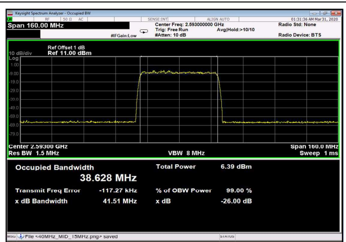
Figure 238: 64QAM 40MHz B.W.; 2593.0MHz, 30kHz Input
