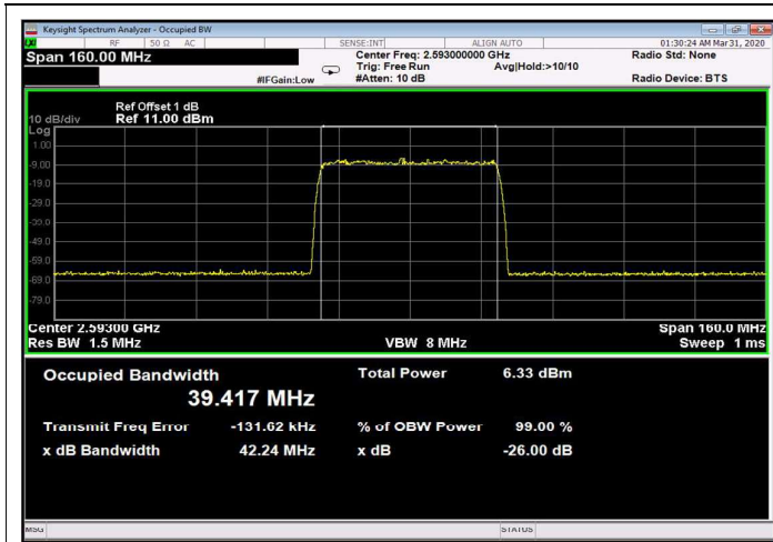
Figure 237: 64QAM 40MHz B.W.; 2593.0MHz, 15kHz Input
