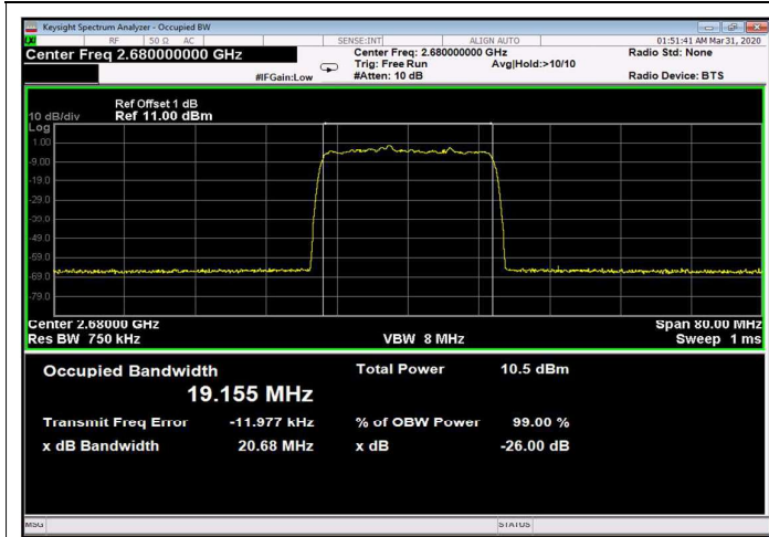
Figure 231: 64QAM 20MHz B.W.; 2680.0MHz, 15kHz Input
