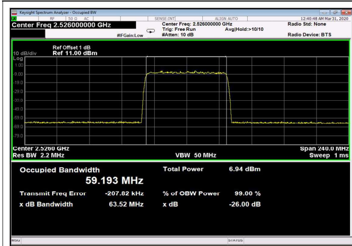
Figure 243: 64QAM 60MHz B.W.; 2526.0MHz, 30kHz Input
