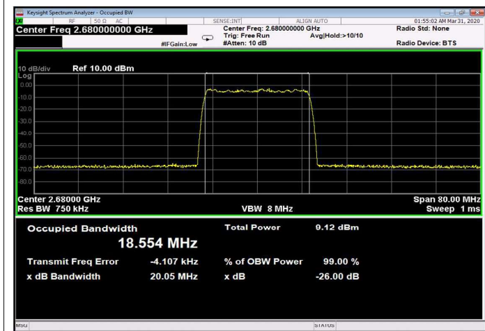
Figure 233: 64QAM 20MHz B.W.; 2680.0MHz, 60kHz Input
