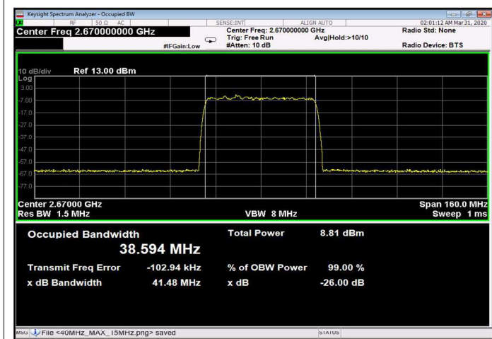
Figure 241: 64QAM 40MHz B.W.; 2670.0MHz, 30kHz Input
