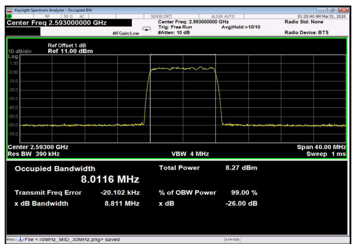
Figure 212: 64QAM 10MHz B.W.; 2593.0MHz, 60kHz Input
