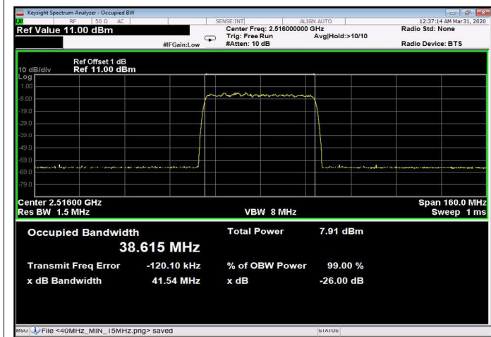
Figure 235: 64QAM 40MHz B.W.; 2516.0MHz, 30kHz Input
