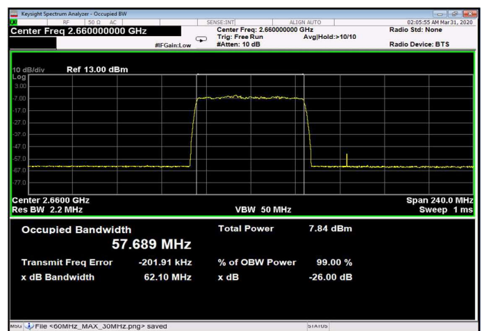
Figure 248: 64QAM 60MHz B.W.; 2660.0MHz, 60kHz Input
