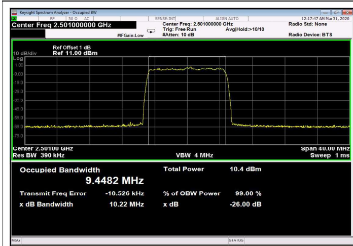
Figure 207: 64QAM 10MHz B.W.; 2501.0MHz, 15kHz Input
