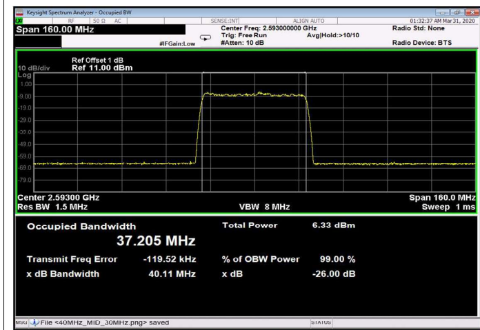
Figure 239: 64QAM 40MHz B.W.; 2593.0MHz, 60kHz Input
