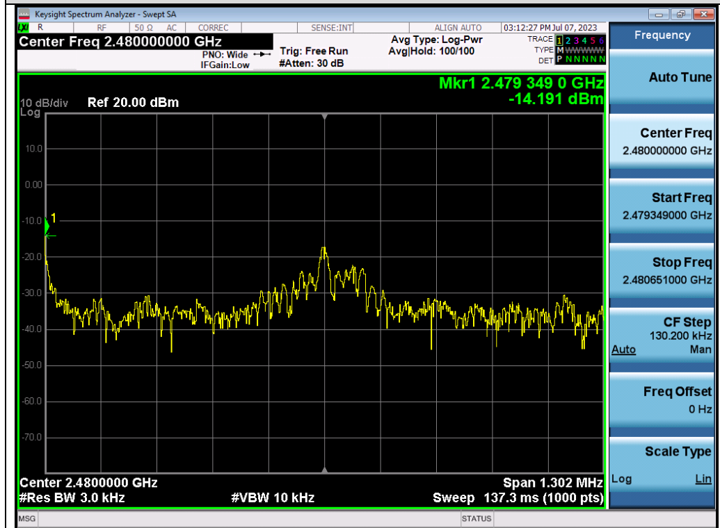
Test_Graph_ANT1_2480_PSD
