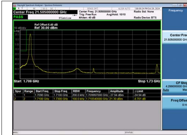
NTNV-n66-PC3-15-20-L-DFT-BPSK-Edge_1RB_Left-PASS
