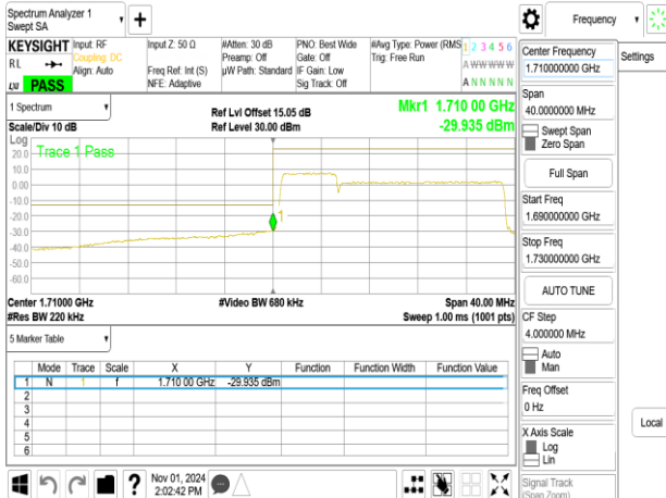
Band66B_5MHz+15MHz_QPSK_RB25-0_75-0_CH132504-132597
