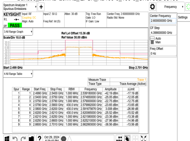
Band41_15MHz+20MHz_QPSK_RB1-0_1-99_CH37928-39899
