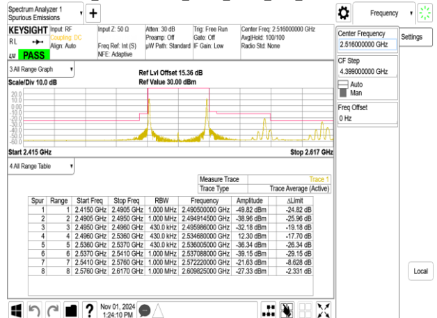
Band41_20MHz+20MHz_QPSK_RB1-0_1-99_CH40521-40719
