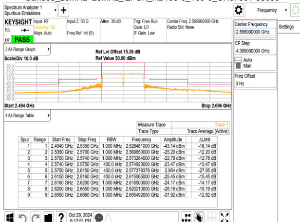
Band38_20MHz+20MHz_QPSK_RB100-0_100-0_CH37901-38099
