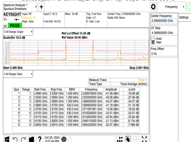
Band38_20MHz+20MHz_QPSK_RB1-0_1-99_CH37901-38099
