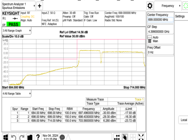
Band12B_5MHz+10MHz_QPSK_RB25-0_50-0_CH23038-23110
