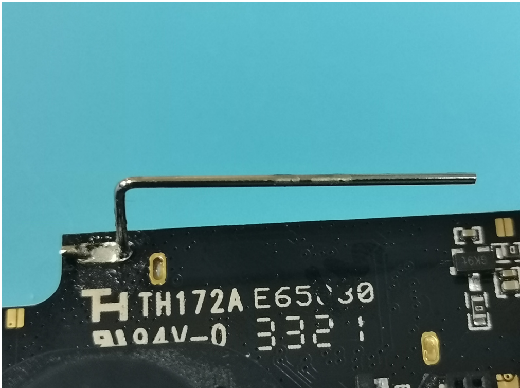
FHSS Antenna
