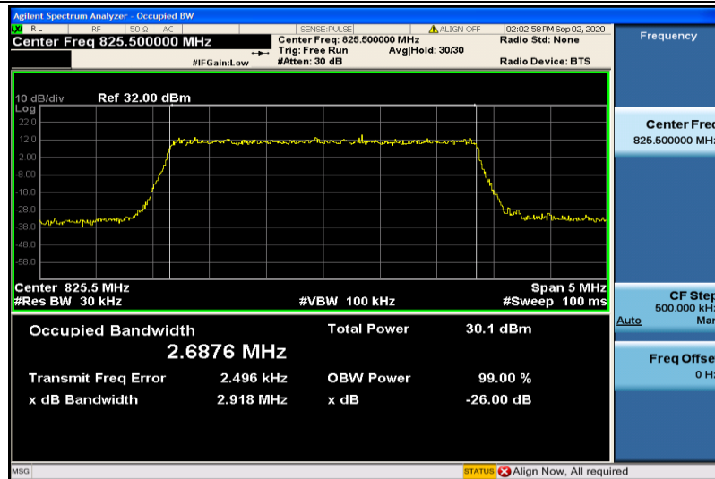
Band5-3MHz-QPSK-20415-15RB#0-2.6876
