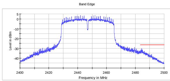
Band Edge Ch08 802.11n HT40 MCS8 MIMO
