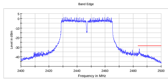
Band Edge Ch08 802.11n HT40 MCS15 MIMO
