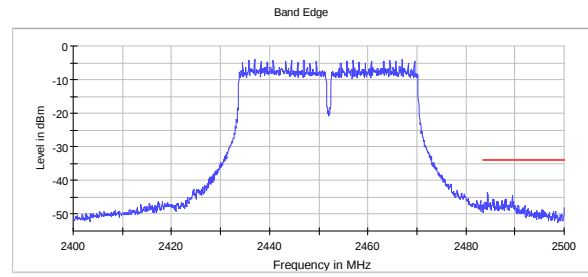
Band Edge Ch09 802.11n HT40 MCS15 MIMO
