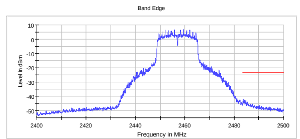
Band Edge
