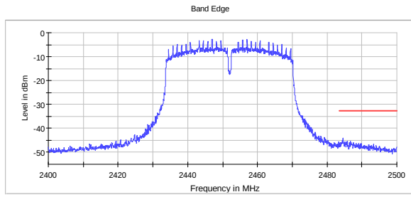
Band Edge Ch09 802.11n HT40 MCS8 MIMO
