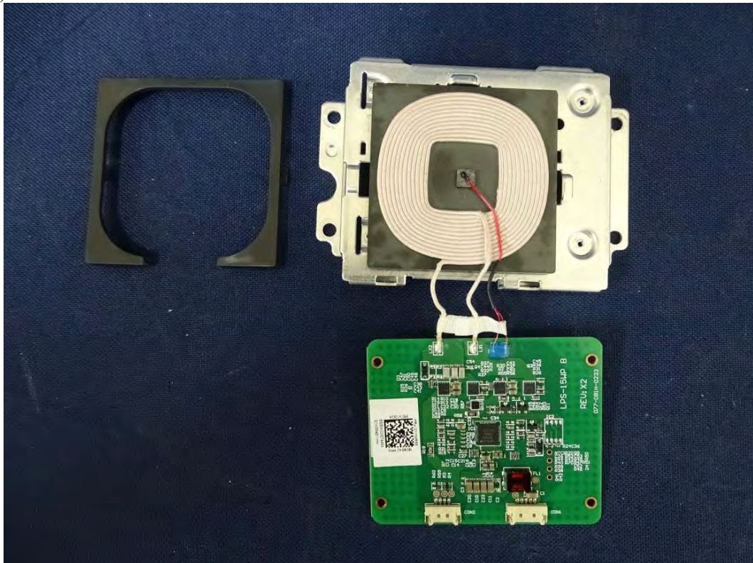
(44) EUT Photo
