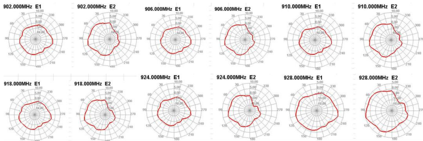
E 面方向图（垂直波瓣方向图）
