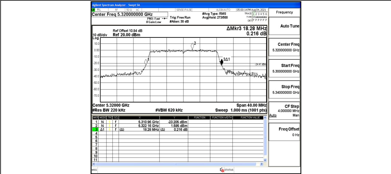
11A_Ant2_5320
