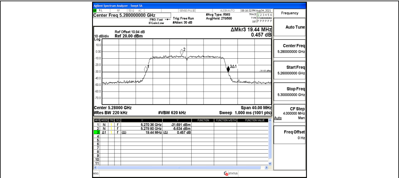
11AC20MIMO_Ant2_5280
