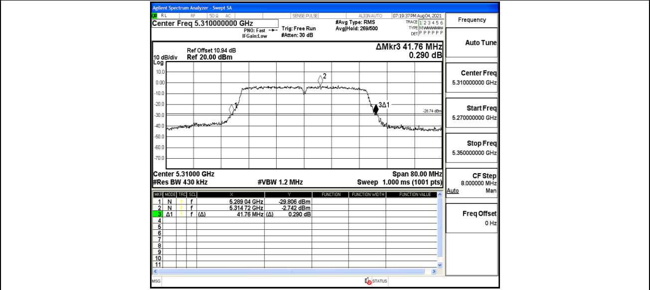
11N40MIMO_Ant2_5310
