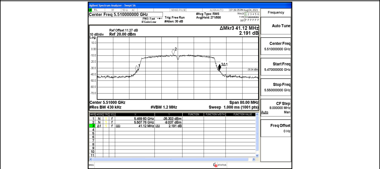
11N40MIMO_Ant2_5510
