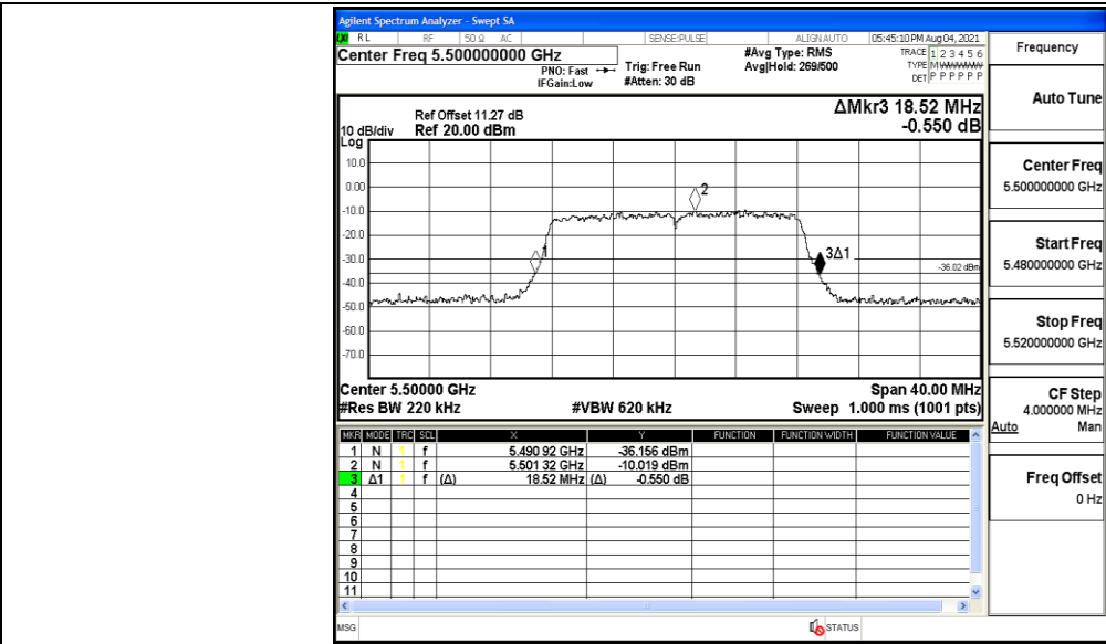
11A_Ant2_5500
