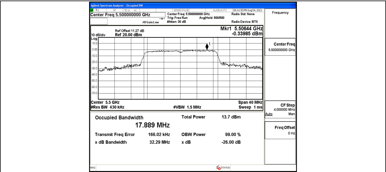
111N20MIMO_Ant2_5500
