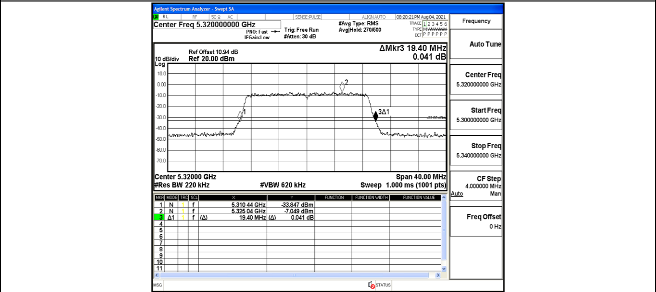
11AC20MIMO_Ant2_5320
