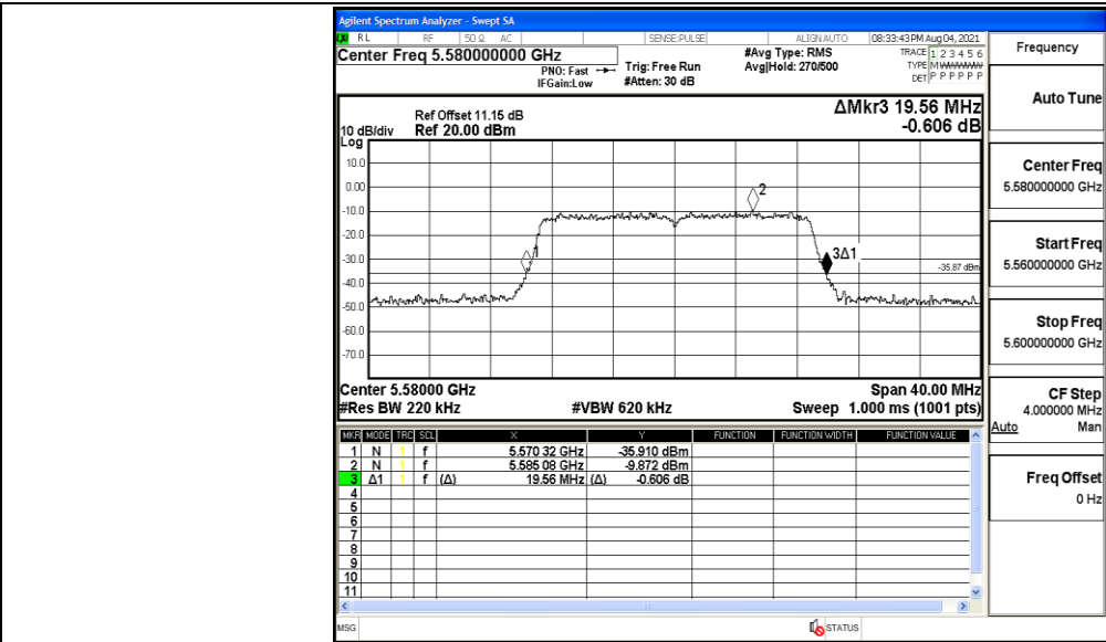
11AC20MIMO_Ant2_5580
