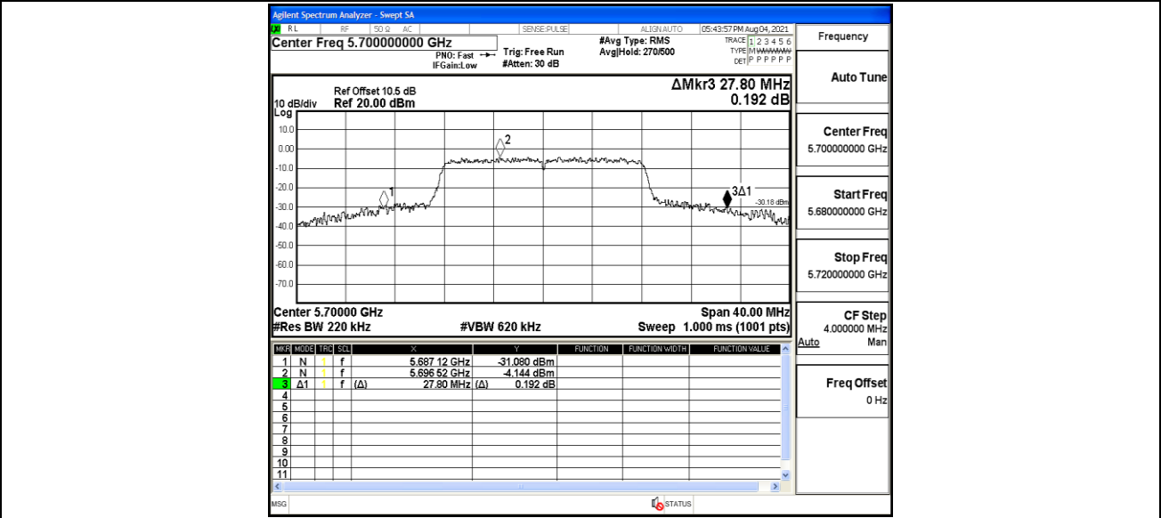
11A_Ant2_5700
