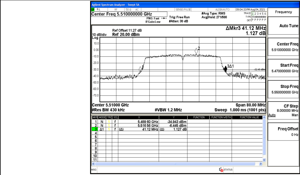
11AC40MIMO_Ant2_5510
