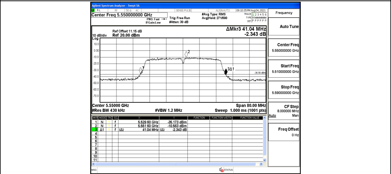
11AC40MIMO_Ant2_5550
