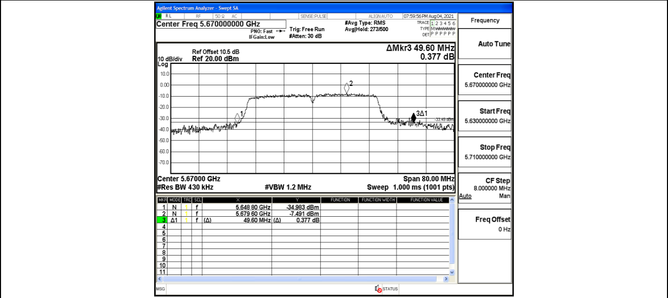
11N40MIMO_Ant2_5670
