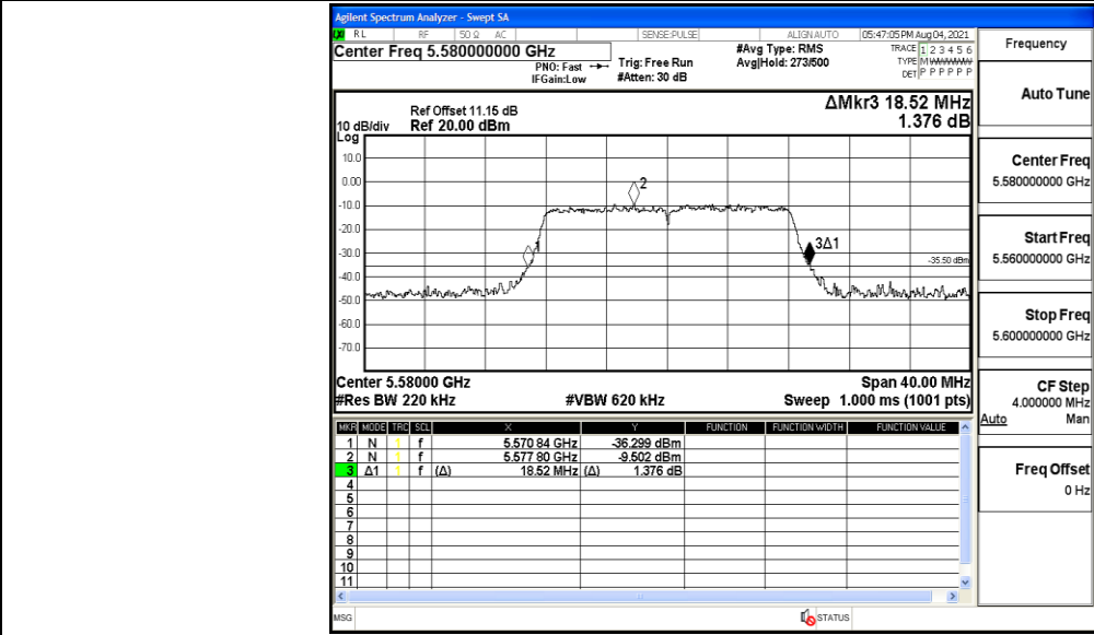
11A_Ant2_5580
