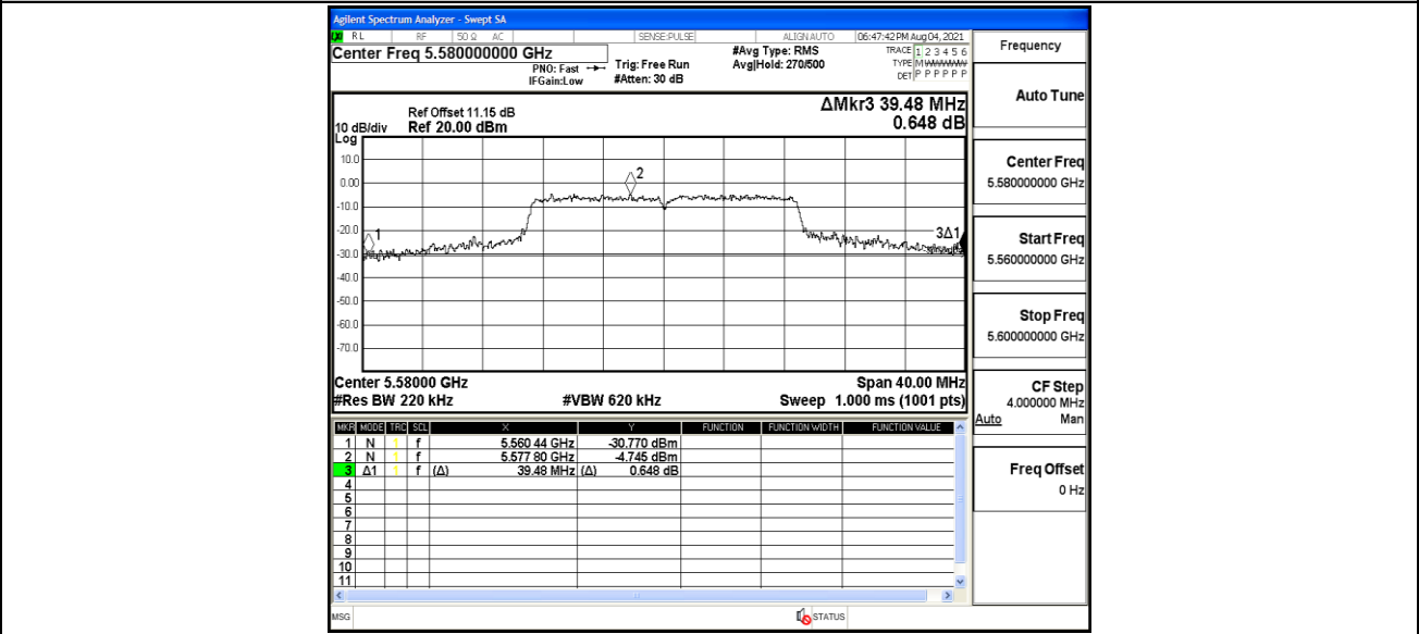
111N20MIMO_Ant2_5580
