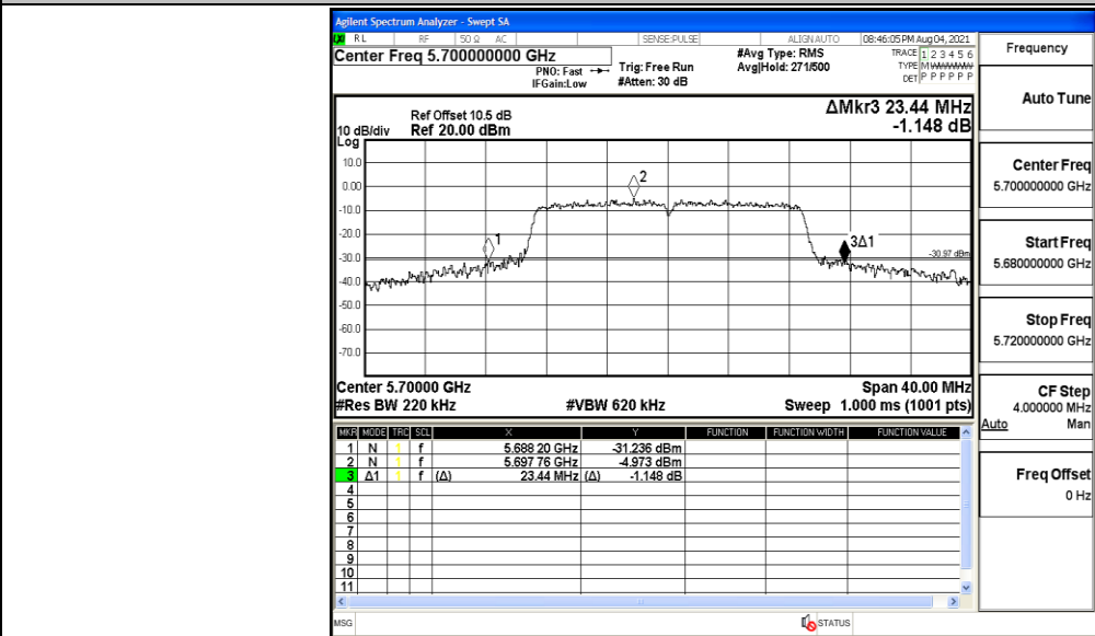
11AC20MIMO_Ant2_5700
