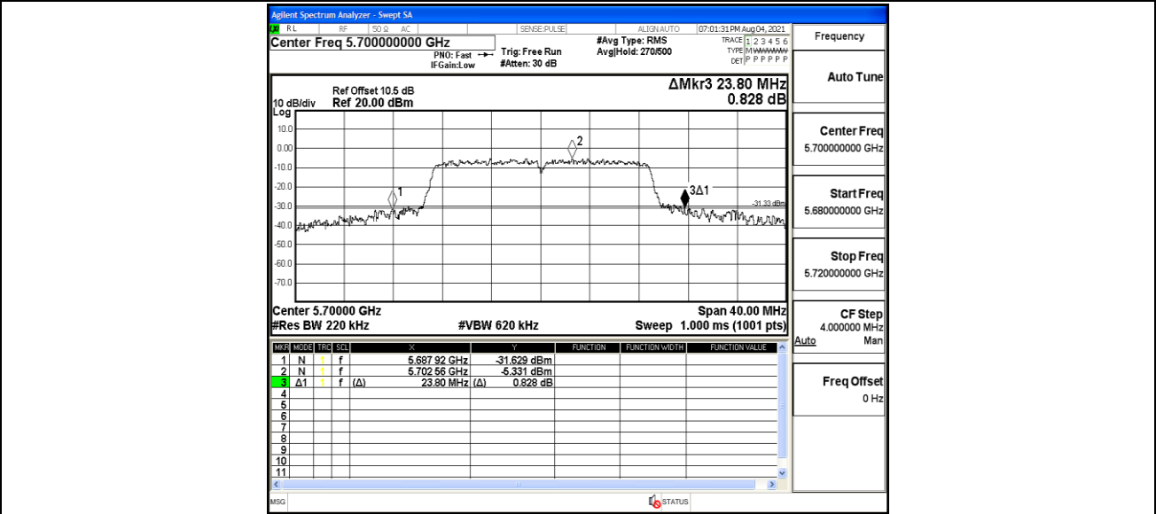
111N20MIMO_Ant2_5700
