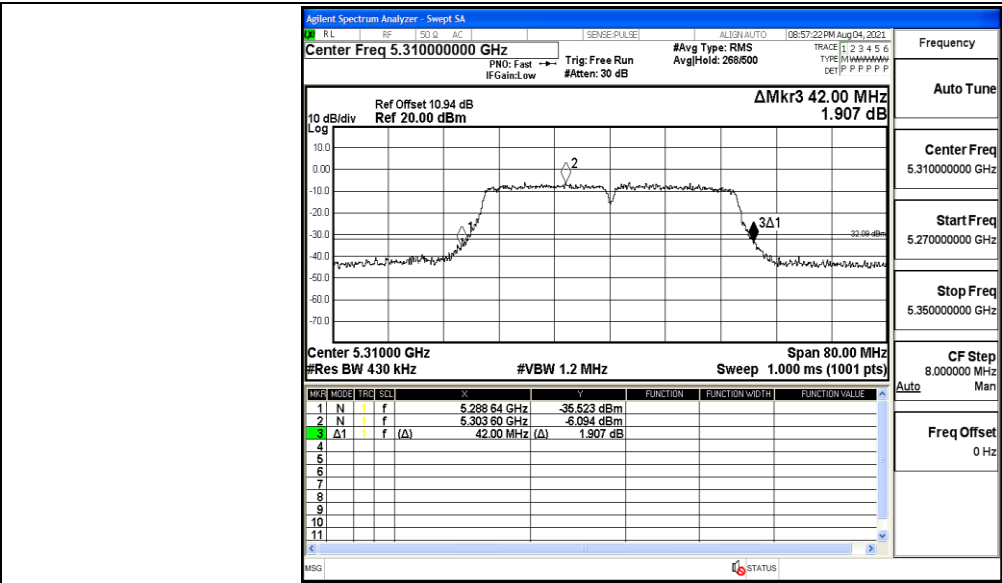
11AC40MIMO_Ant2_5310
