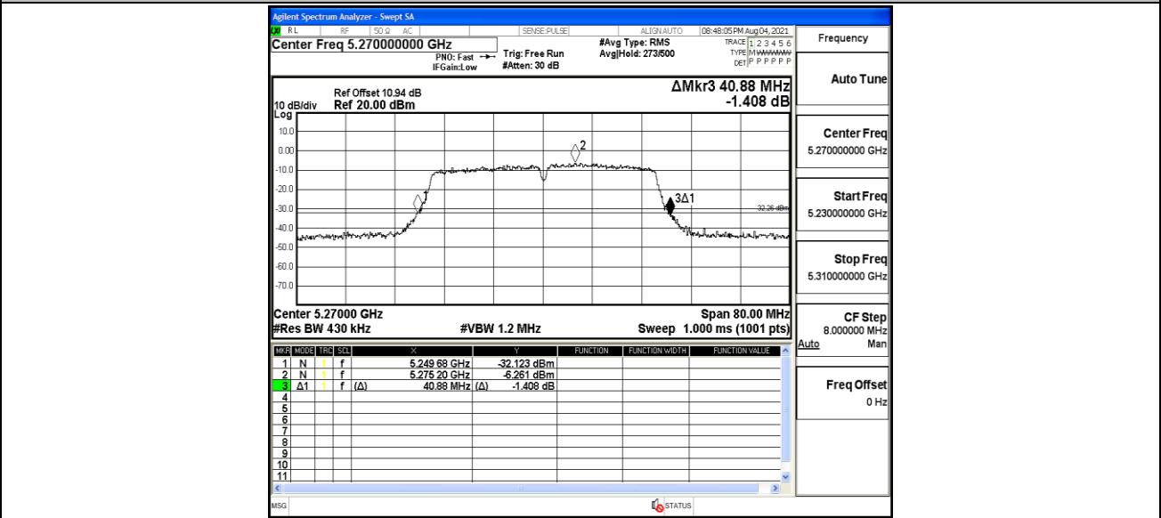
11AC40MIMO_Ant2_5270
