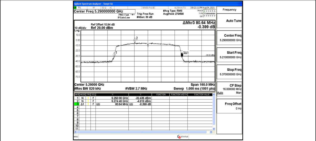
11AC80MIMO_Ant2_5290
