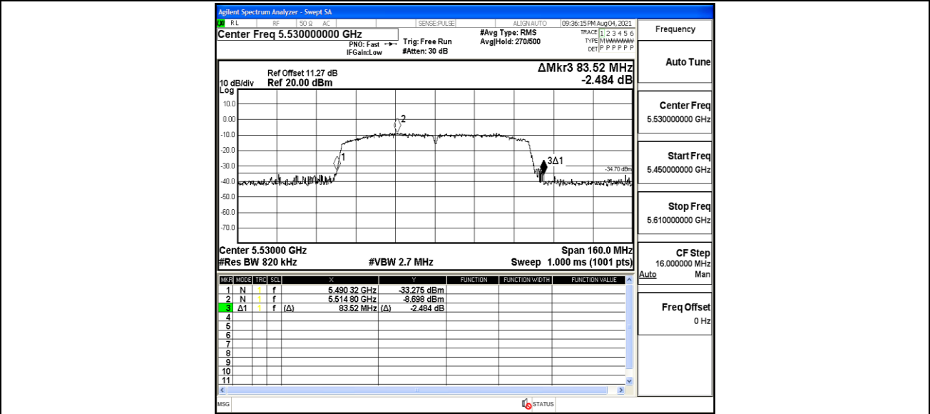
11AC80MIMO_Ant2_5530
