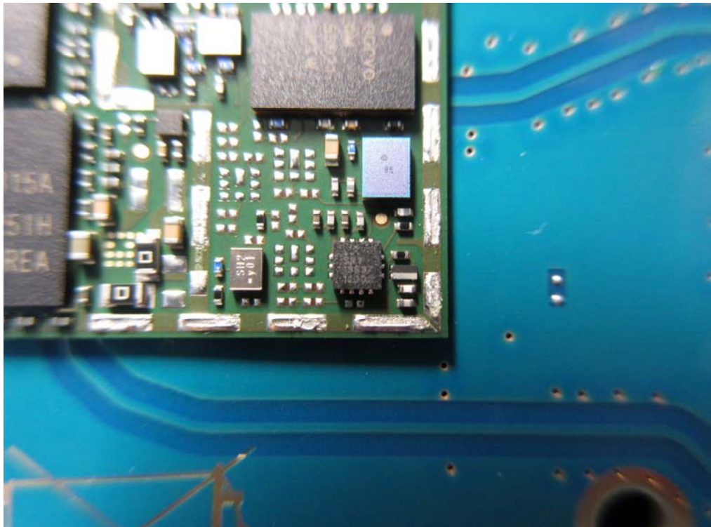
(13) EUT Photo
