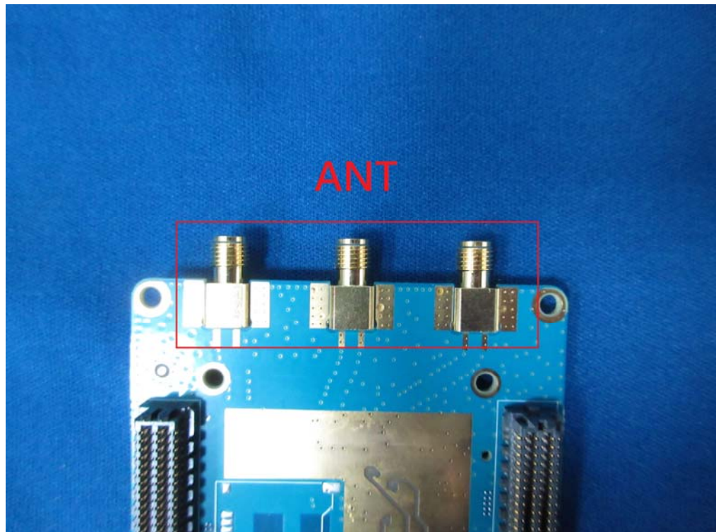
(18) EUT Photo (Antenna)
