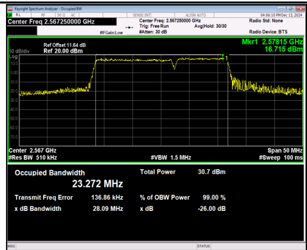
41(2555-2655)-41(2555-2655)-15MHz-10MHz-16QAM-16Q AM-40315-40435-75RB#0-50RB#0-PASS
