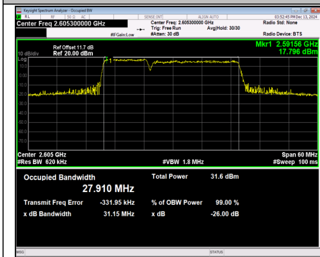
41(2555-2655)-41(2555-2655)-10MHz-20MHz-QPSK-QP SK-40646-40790-50RB#0-100RB#0-PASS
