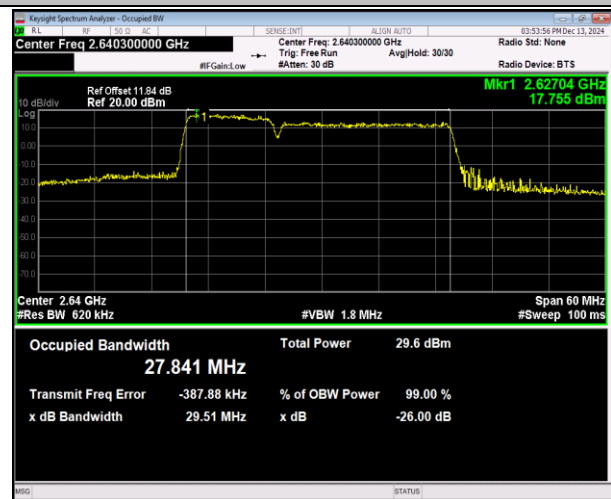
41(2555-2655)-41(2555-2655)-10MHz-20MHz-16QAM-16Q AM-40996-41140-50RB#0-100RB#0-PASS
