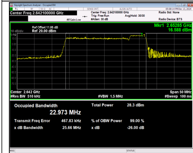
41(2555-2655)-41(2555-2655)-20MHz-5MHz-QPSK-QPS K-41090-41207-100RB#0-25RB#0-PASS
