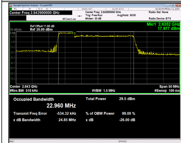
41(2555-2655)-41(2555-2655)-5MHz-20MHz-QPSK-QPS K-41023-41140-25RB#0-100RB#0-PASS
