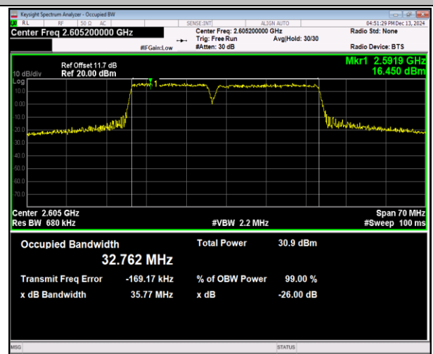
41(2555-2655)-41(2555-2655)-15MHz-20MHz-16QAM-16Q AM-40644-40815-75RB#0-100RB#0-PASS
