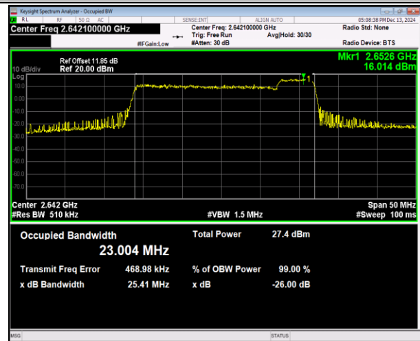
41(2555-2655)-41(2555-2655)-20MHz-5MHz-16QAM-16QA M-41090-41207-100RB#0-25RB#0-PASS
