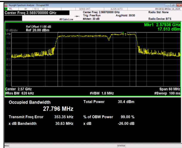
41(2555-2655)-41(2555-2655)-20MHz-10MHz-16QAM-16Q AM-40340-40484-100RB#0-50RB#0-PASS
