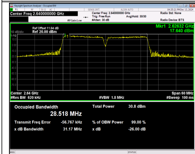
41(2555-2655)-41(2555-2655)-15MHz-15MHz-QPSK-QP SK-41015-41165-75RB#0-75RB#0-PASS
