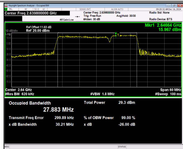
41(2555-2655)-41(2555-2655)-20MHz-10MHz-16QAM-16Q AM-41041-41185-100RB#0-50RB#0-PASS
