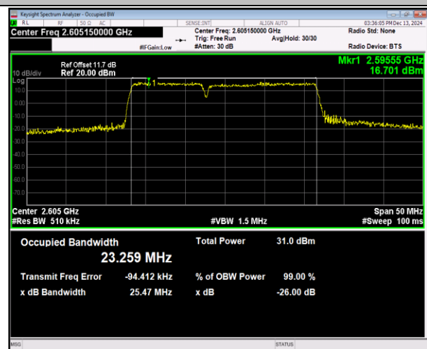
41(2555-2655)-41(2555-2655)-10MHz-15MHz-16QAM-16Q AM-40669-40789-50RB#0-75RB#0-PASS
