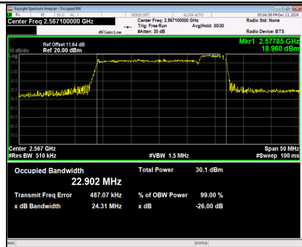
41(2555-2655)-41(2555-2655)-20MHz-5MHz-16QAM-16QA M-40340-40457-100RB#0-25RB#0-PASS
