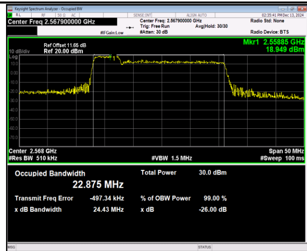
41(2555-2655)-41(2555-2655)-5MHz-20MHz-16QAM-16QA M-40273-40390-25RB#0-100RB#0-PASS
