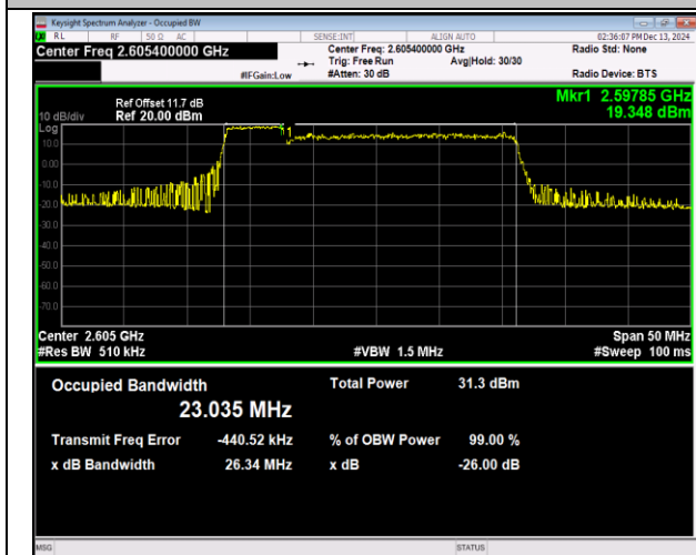
41(2555-2655)-41(2555-2655)-5MHz-20MHz-QPSK-QPS K-40648-40765-25RB#0-100RB#0-PASS
