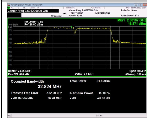
41(2555-2655)-41(2555-2655)-15MHz-20MHz-QPSK-QP SK-40644-40815-75RB#0-100RB#0-PASS
