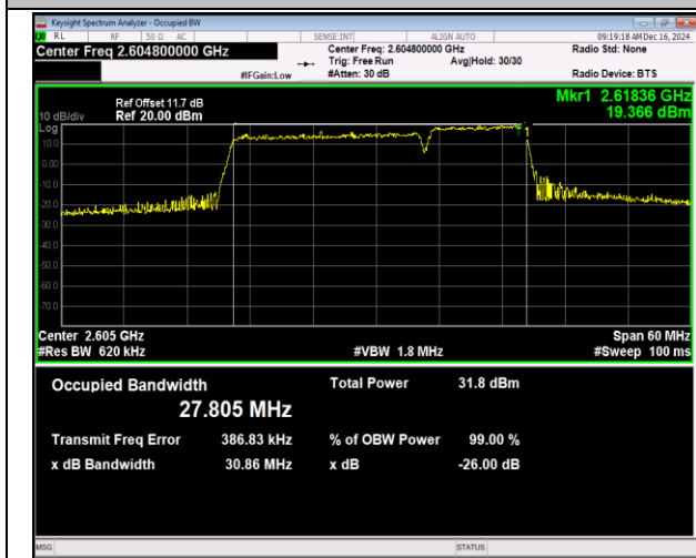
41(2555-2655)-41(2555-2655)-20MHz-10MHz-QPSK-QP SK-40691-40835-100RB#0-50RB#0-PASS
