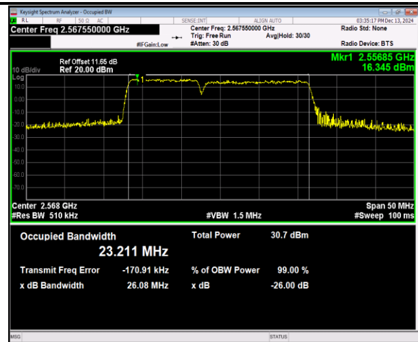
41(2555-2655)-41(2555-2655)-10MHz-15MHz-16QAM-16Q AM-40293-40413-50RB#0-75RB#0-PASS
