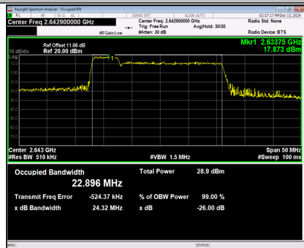
41(2555-2655)-41(2555-2655)-5MHz-20MHz-16QAM-16QA M-41023-41140-25RB#0-100RB#0-PASS
