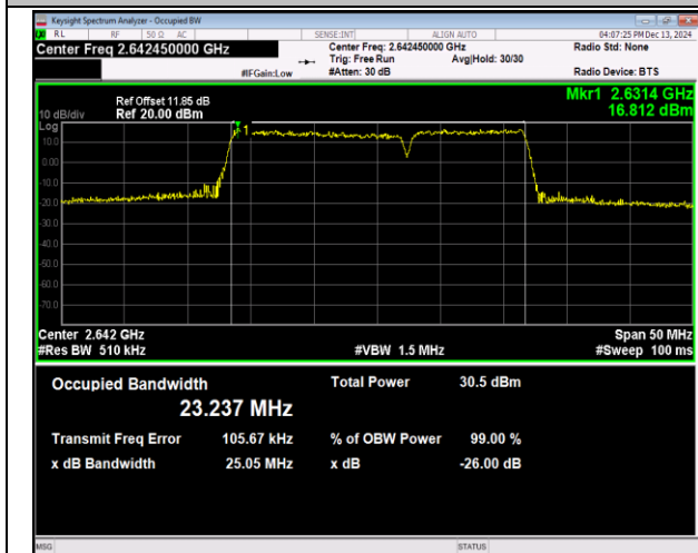
41(2555-2655)-41(2555-2655)-15MHz-10MHz-QPSK-QP SK-41067-41187-75RB#0-50RB#0-PASS
