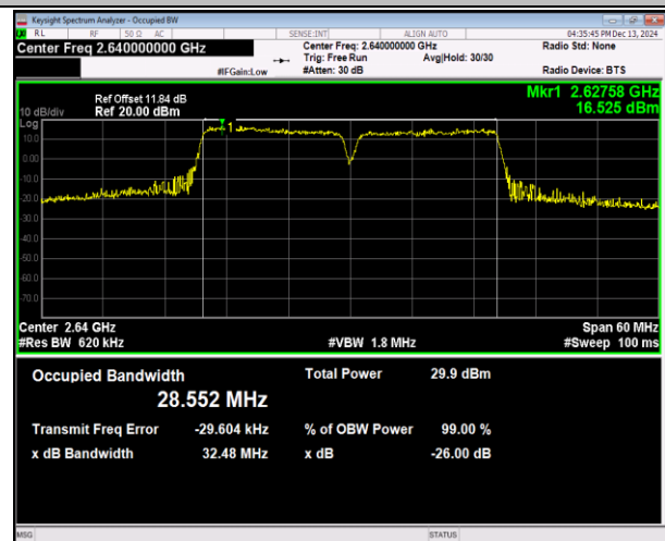
41(2555-2655)-41(2555-2655)-15MHz-15MHz-16QAM-16Q AM-41015-41165-75RB#0-75RB#0-PASS
