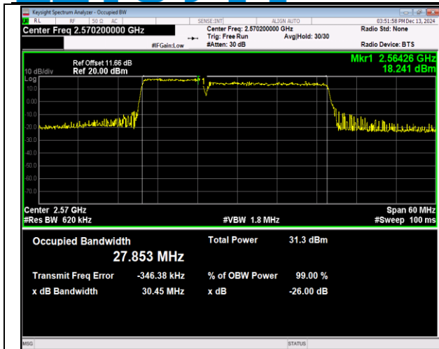
41(2555-2655)-41(2555-2655)-10MHz-20MHz-QPSK-QP SK-40295-40439-50RB#0-100RB#0-PASS
