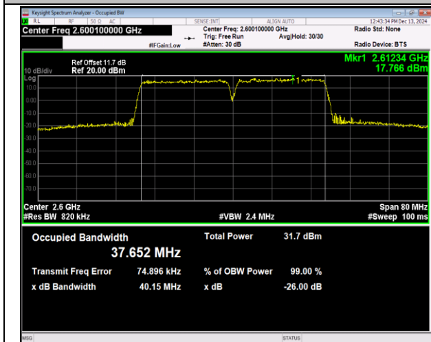
38-38-20MHz-20MHz-QPSK-QPSK-37952-38150-100RB #0-100RB#0-PASS
