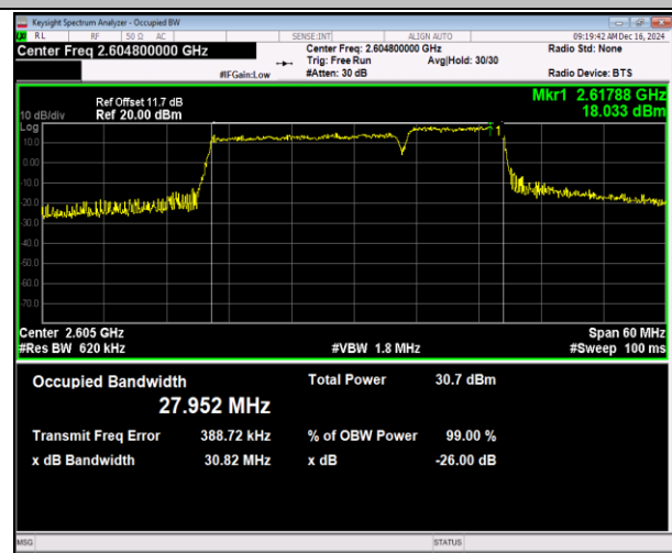
41(2555-2655)-41(2555-2655)-20MHz-10MHz-16QAM-16Q AM-40691-40835-100RB#0-50RB#0-PASS
