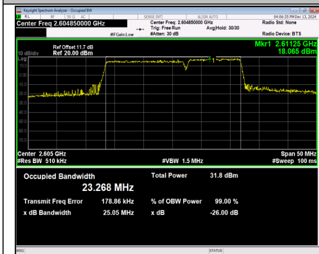
41(2555-2655)-41(2555-2655)-15MHz-10MHz-QPSK-QP SK-40691-40811-75RB#0-50RB#0-PASS
