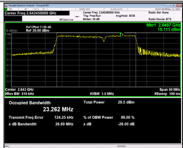
41(2555-2655)-41(2555-2655)-15MHz-10MHz-16QAM-16Q AM-41067-41187-75RB#0-50RB#0-PASS
