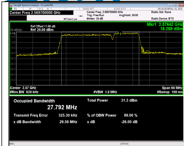
41(2555-2655)-41(2555-2655)-20MHz-10MHz-QPSK-QP SK-40340-40484-100RB#0-50RB#0-PASS
