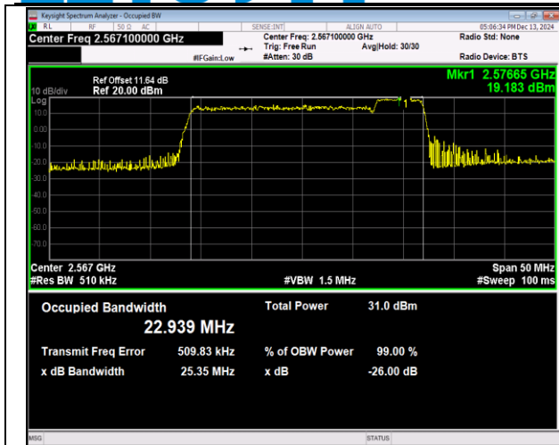
41(2555-2655)-41(2555-2655)-20MHz-5MHz-QPSK-QPS K-40340-40457-100RB#0-25RB#0-PASS
