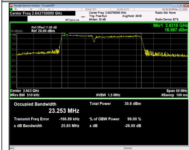
41(2555-2655)-41(2555-2655)-10MHz-15MHz-QPSK-QP SK-41045-41165-50RB#0-75RB#0-PASS
