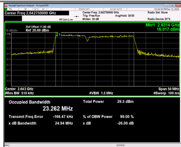
41(2555-2655)-41(2555-2655)-10MHz-15MHz-16QAM-16Q AM-41045-41165-50RB#0-75RB#0-PASS
