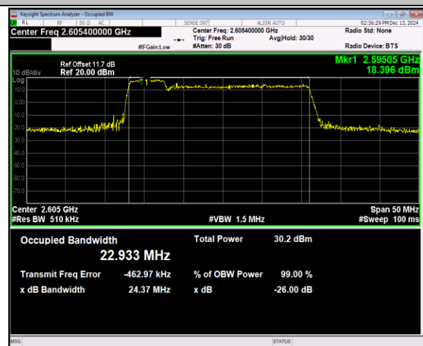
41(2555-2655)-41(2555-2655)-5MHz-20MHz-16QAM-16QA M-40648-40765-25RB#0-100RB#0-PASS
