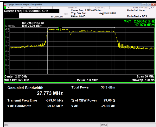
41(2555-2655)-41(2555-2655)-10MHz-20MHz-16QAM-16Q AM-40295-40439-50RB#0-100RB#0-PASS
