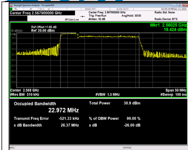
41(2555-2655)-41(2555-2655)-5MHz-20MHz-QPSK-QPS K-40273-40390-25RB#0-100RB#0-PASS
