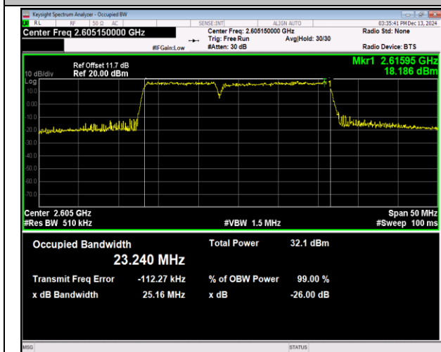
41(2555-2655)-41(2555-2655)-10MHz-15MHz-QPSK-QP SK-40669-40789-50RB#0-75RB#0-PASS
