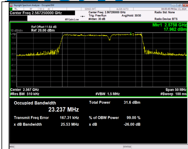
41(2555-2655)-41(2555-2655)-15MHz-10MHz-QPSK-QP SK-40315-40435-75RB#0-50RB#0-PASS
