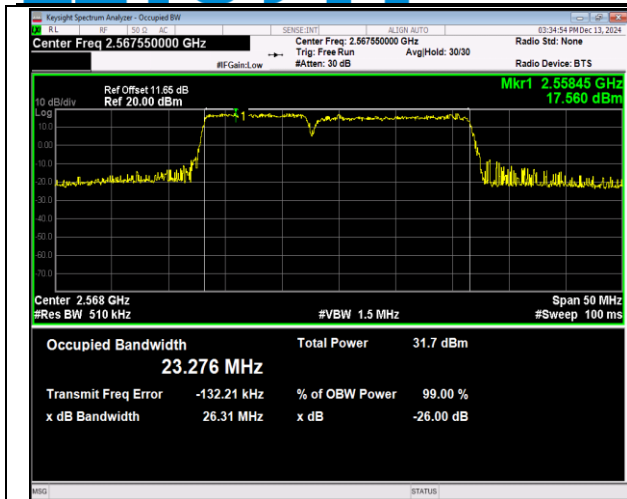
41(2555-2655)-41(2555-2655)-10MHz-15MHz-QPSK-QP SK-40293-40413-50RB#0-75RB#0-PASS
