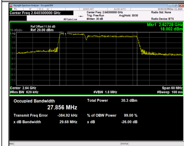
41(2555-2655)-41(2555-2655)-10MHz-20MHz-QPSK-QP SK-40996-41140-50RB#0-100RB#0-PASS
