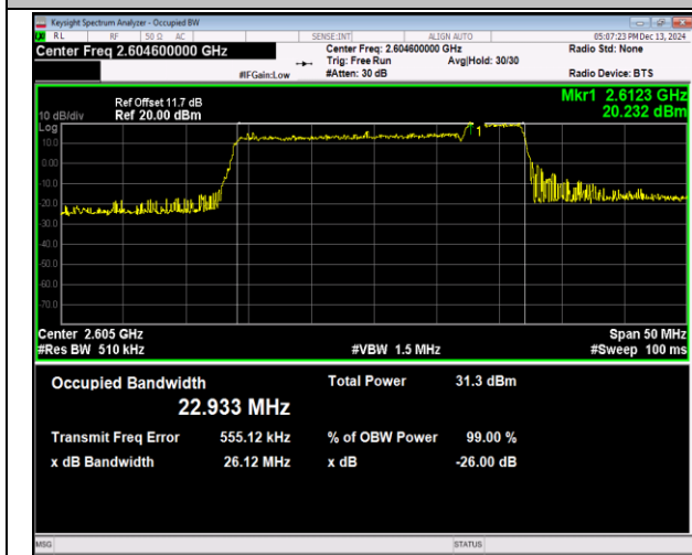
41(2555-2655)-41(2555-2655)-20MHz-5MHz-QPSK-QPS K-40715-40832-100RB#0-25RB#0-PASS
