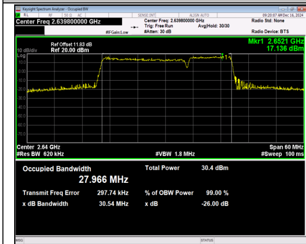
41(2555-2655)-41(2555-2655)-20MHz-10MHz-QPSK-QP SK-41041-41185-100RB#0-50RB#0-PASS
