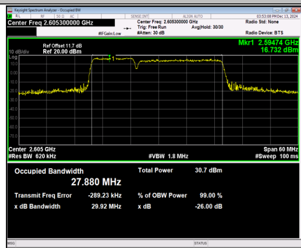
41(2555-2655)-41(2555-2655)-10MHz-20MHz-16QAM-16Q AM-40646-40790-50RB#0-100RB#0-PASS
