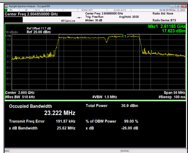
41(2555-2655)-41(2555-2655)-15MHz-10MHz-16QAM-16Q AM-40691-40811-75RB#0-50RB#0-PASS
