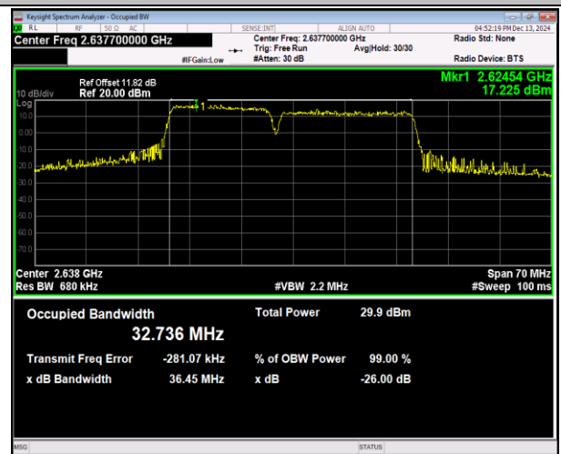
41(2555-2655)-41(2555-2655)-15MHz-20MHz-16QAM-16Q AM-40969-41140-75RB#0-100RB#0-PASS
