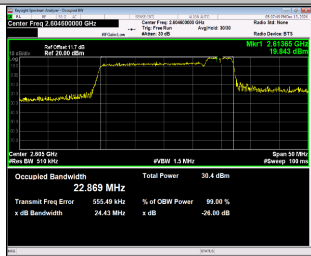
41(2555-2655)-41(2555-2655)-20MHz-5MHz-16QAM-16QA M-40715-40832-100RB#0-25RB#0-PASS
