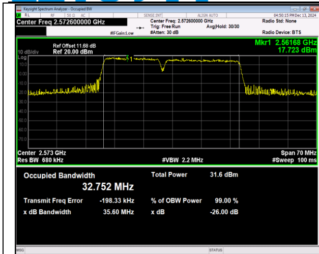
41(2555-2655)-41(2555-2655)-15MHz-20MHz-QPSK-QP SK-40318-40489-75RB#0-100RB#0-PASS
