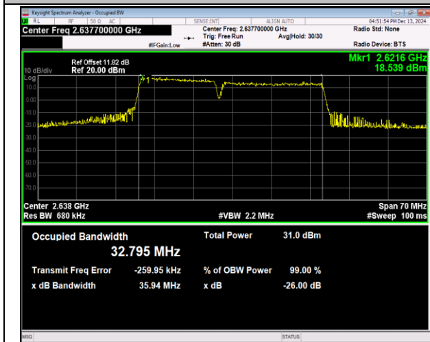
41(2555-2655)-41(2555-2655)-15MHz-20MHz-QPSK-QP SK-40969-41140-75RB#0-100RB#0-PASS
