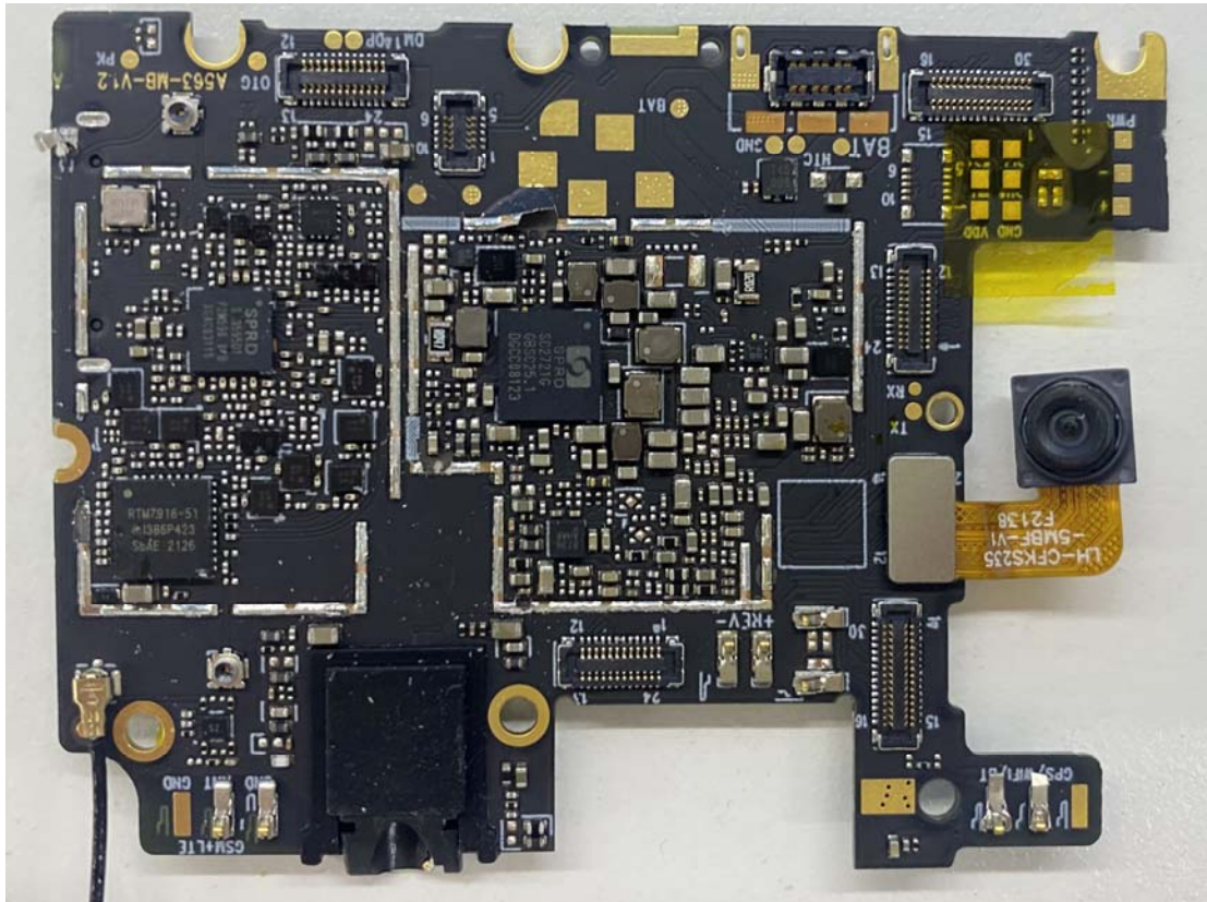
IC Details 1
