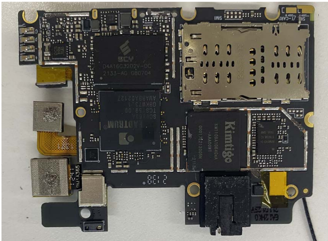
IC Details 4
