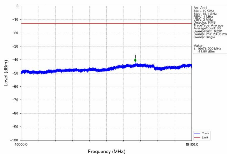
Band2_10MHz_QPSK_HCH_1905MHz_RB_1_49_NTNV
