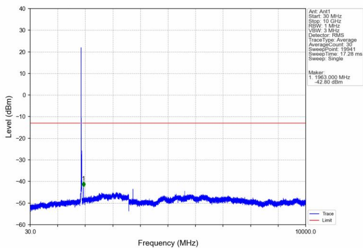
Band2_15MHz_QPSK_MCH_1880MHz_RB_1_0_NTNV
