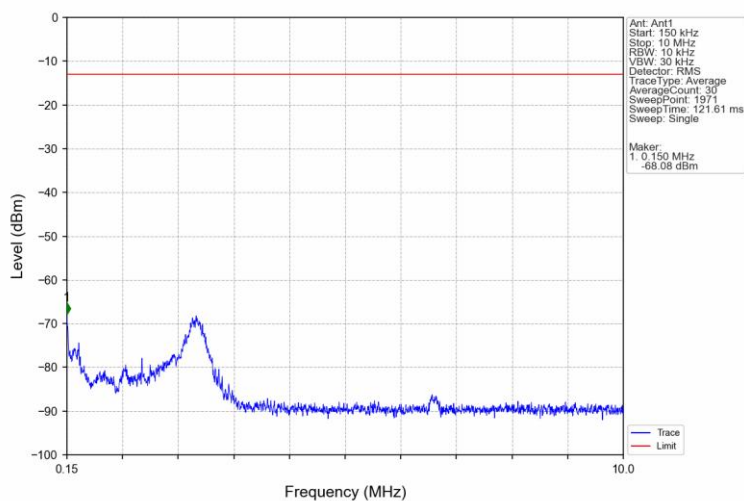
Band2_15MHz_QPSK_HCH_1902.5MHz_RB_1_0_NTNV
