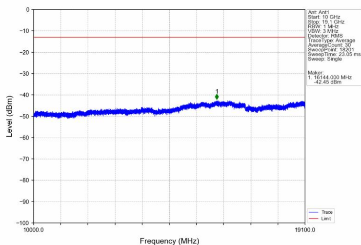
Band2_15MHz_QPSK_HCH_1902.5MHz_RB_1_74_NTNV
