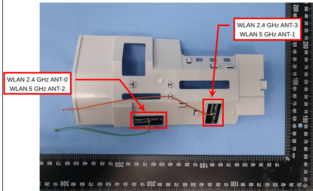
EUT Photo (4)
