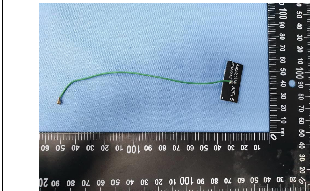
EUT Photo (4)
