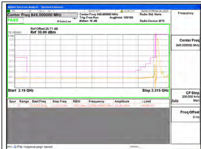
Band30 / 5MHz / Low CH / QPSK / 1 RB
