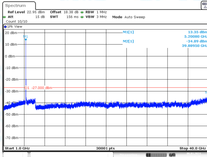
11N20-CDD_Ant1_5200_1000~40000
