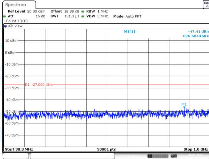
11N40-CDD_Ant1_5190_30~1000
