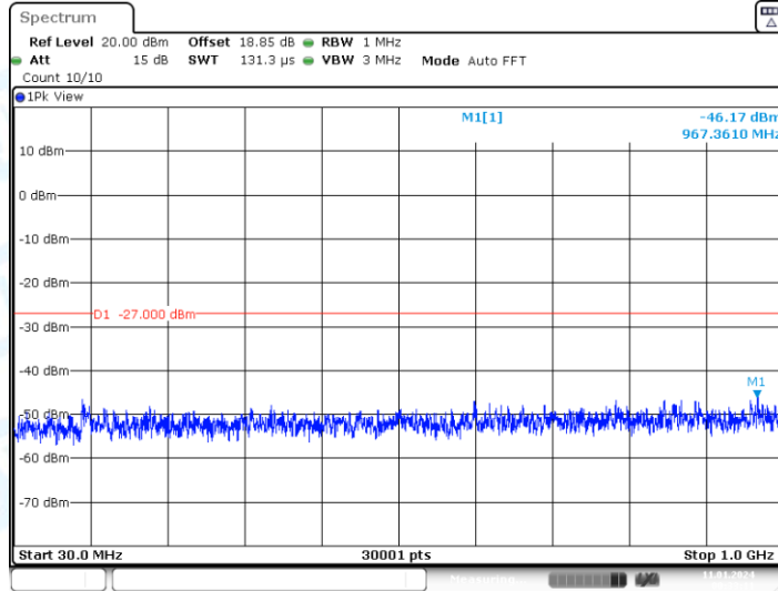
11A-CDD_Ant2_5720_30~1000
