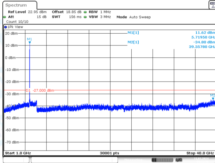
11A-CDD_Ant2_5720_1000~40000
