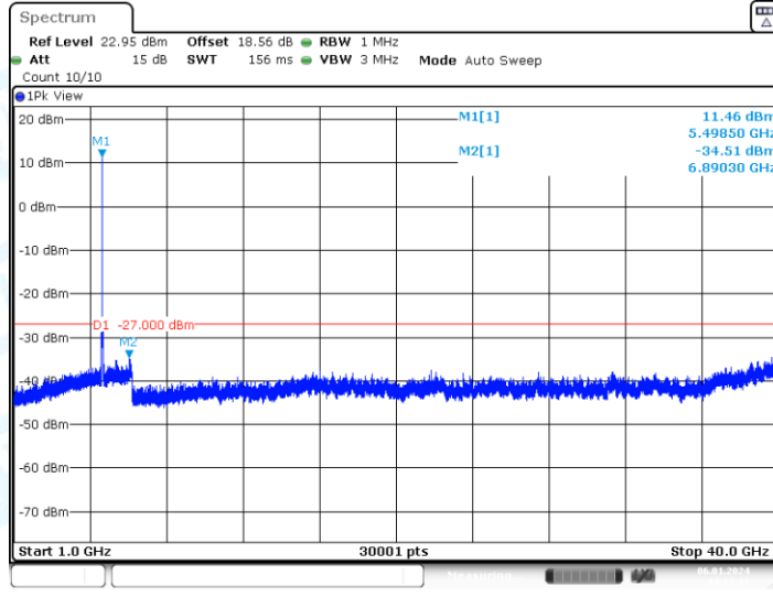
11N20-CDD_Ant1_5500_1000~40000
