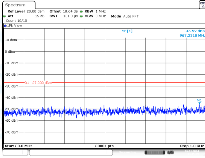
11N20-CDD_Ant2_5500_30~1000
