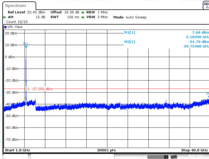
11N40-CDD_Ant1_5190_1000~40000
