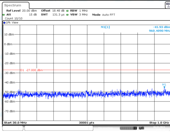
11N40-CDD_Ant1_5230_30~1000
