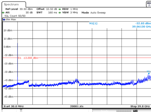
n77_3_20MHz_30kHz_3970MHz_DFT-s-OFDM QPSK_RB50@0 -32.85dBm
