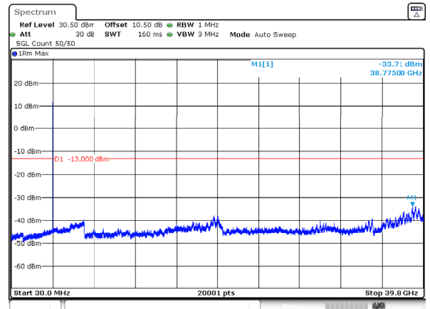
n77_3_20MHz_30kHz_3970MHz_DFT-s-OFDM QPSK_RB1@50 -33.71dBm
