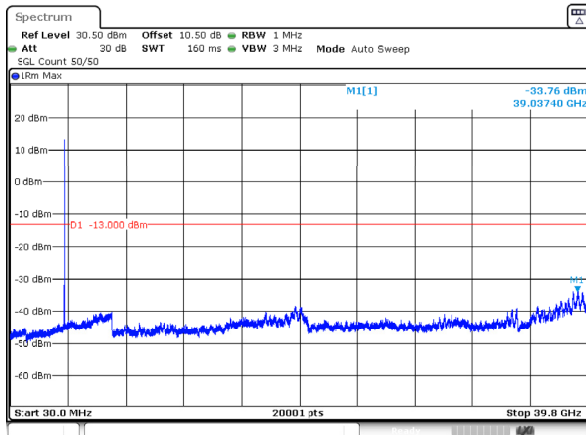
n77_3_40MHz_30kHz_3720MHz_DFT-s-OFDM QPSK_RB1@105 -33.76dBm
