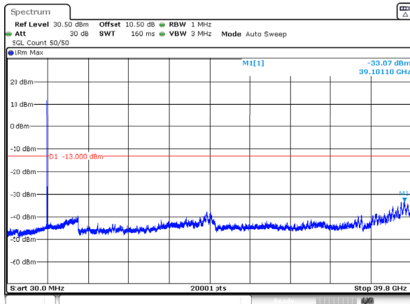
n77_3_80MHz_30kHz_3940MHz_DFT-s-OFDM QPSK_RB1@0 -33.07dBm
