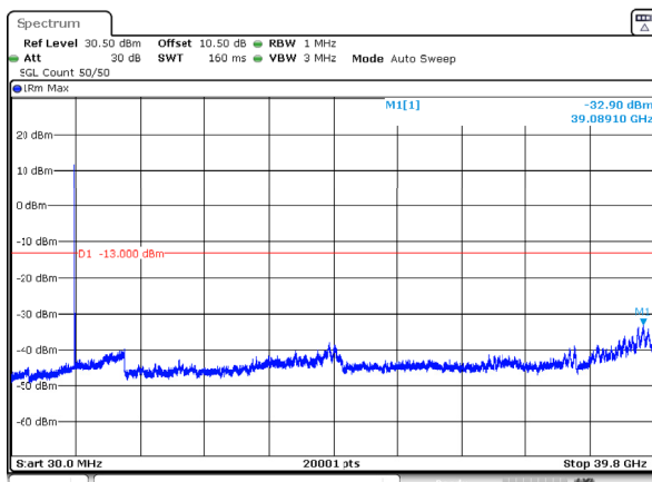
n77_3_50MHz_30kHz_3955MHz_DFT-s-OFDM QPSK_RB1@0 -32.90dBm
