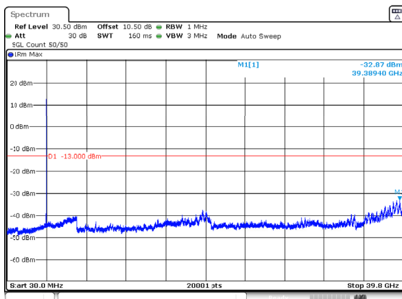
n77_3_90MHz_30kHz_3935MHz_DFT-s-OFDM QPSK_RB1@244 -32.87dBm
