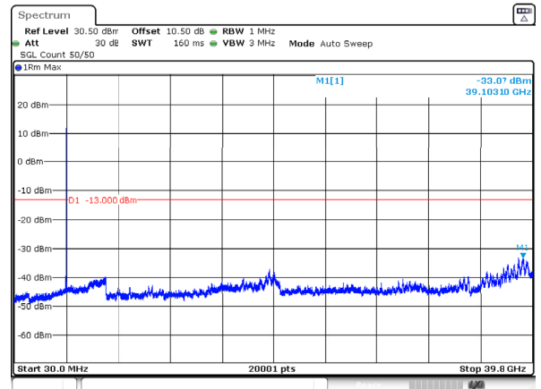
n77_3_80MHz_30kHz_3940MHz_DFT-s-OFDM QPSK_RB1@216 -33.07dBm
