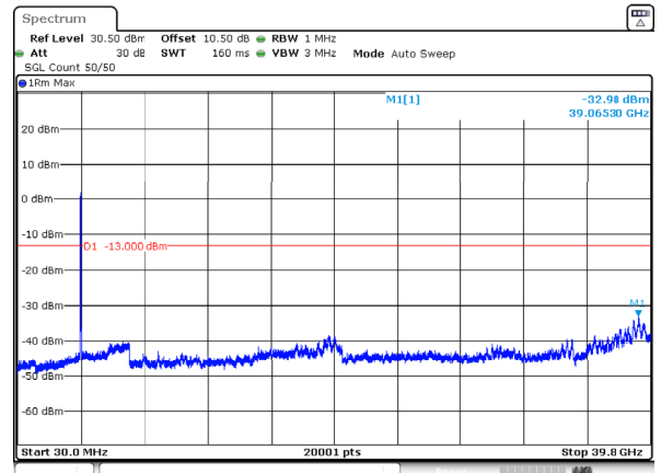
n77_3_50MHz_30kHz_3955MHz_DFT-s-OFDM QPSK_RB128@0 -32.98dBm
