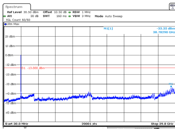
n77_3_60MHz_30kHz_3950MHz_DFT-s-OFDM QPSK_RB162@0 -33.35dBm
