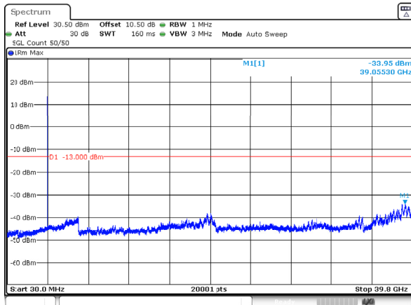
n77_3_20MHz_30kHz_3970MHz_DFT-s-OFDM QPSK_RB1@0 -33.95dBm
