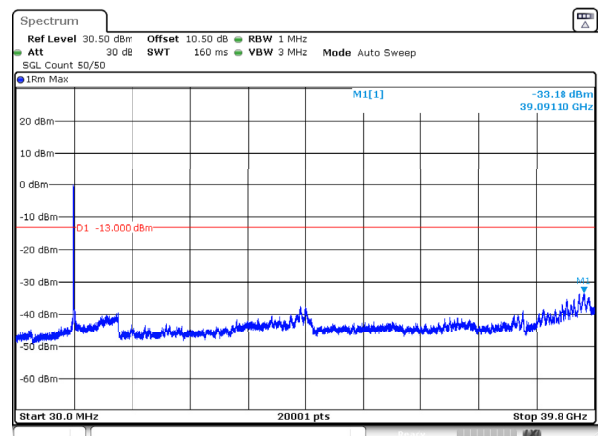
n77_3_90MHz_30kHz_3935MHz_DFT-s-OFDM QPSK_RB243@0 -33.18dBm
