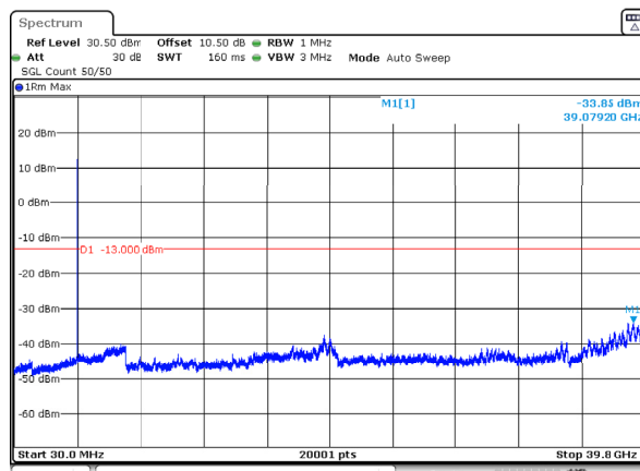
n77_3_30MHz_30kHz_3965MHz_DFT-s-OFDM QPSK_RB1@0 -33.85dBm
