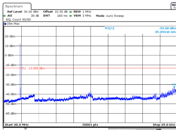
n77_3_60MHz_30kHz_3730MHz_DFT-s-OFDM QPSK_RB1@0 -33.60dBm
