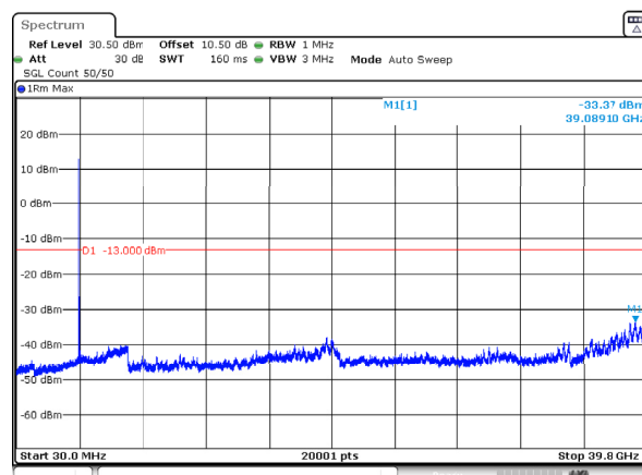
n77_3_60MHz_30kHz_3950MHz_DFT-s-OFDM QPSK_RB1@0 -33.37dBm
