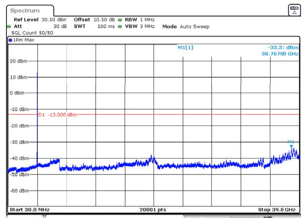
n77_3_50MHz_30kHz_3955MHz_DFT-s-OFDM QPSK_RB1@132 -33.31dBm
