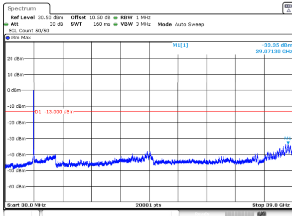
n77_3_80MHz_30kHz_3940MHz_DFT-s-OFDM QPSK_RB216@0 -33.35dBm
