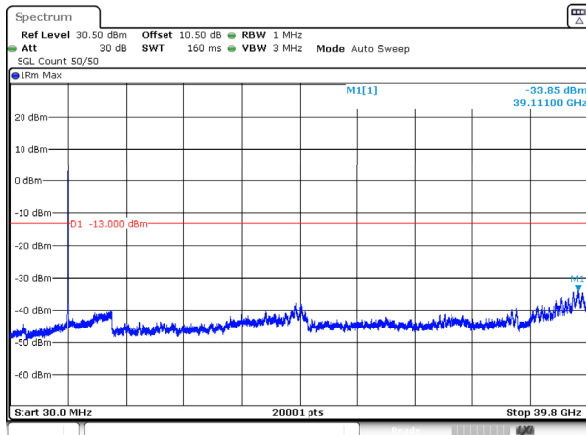
n77_3_40MHz_30kHz_3960MHz_DFT-s-OFDM QPSK_RB100@0 -33.85dBm
