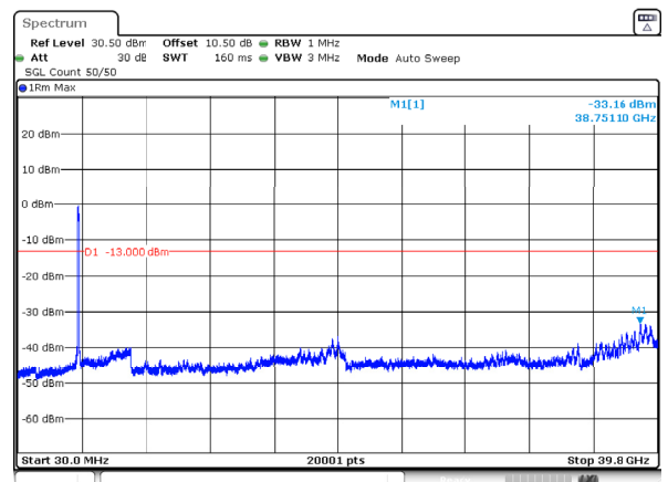
n77_3_90MHz_30kHz_3745MHz_DFT-s-OFDM QPSK_RB243@0 -33.16dBm
