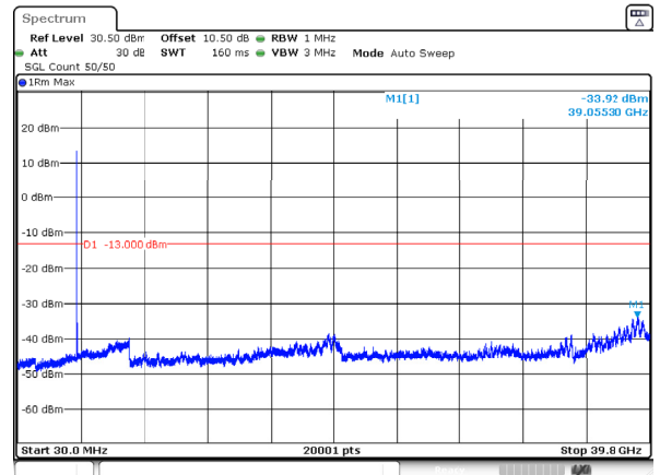
n77_3_40MHz_30kHz_3720MHz_DFT-s-OFDM QPSK_RB1@0 -33.92dBm
