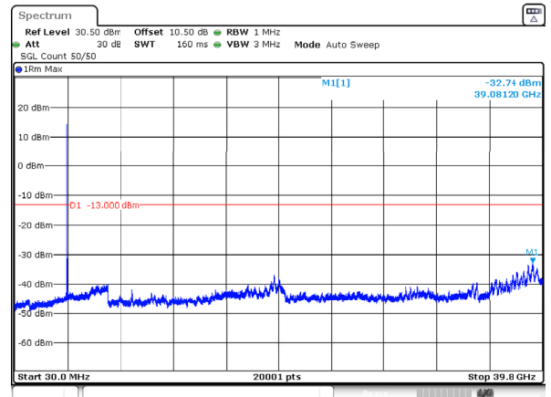
n77_3_90MHz_30kHz_3935MHz_DFT-s-OFDM QPSK_RB1@0 -32.74dBm
