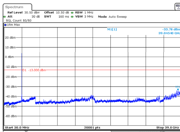
n77_3_30MHz_30kHz_3965MHz_DFT-s-OFDM QPSK_RB75@0 -33.78dBm
