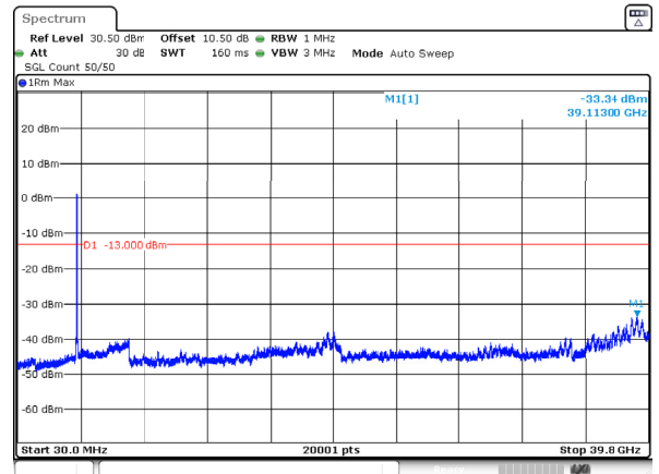
n77_3_50MHz_30kHz_3725MHz_DFT-s-OFDM QPSK_RB128@0 -33.34dBm
