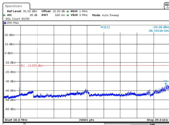
n77_3_80MHz_30kHz_3740MHz_DFT-s-OFDM QPSK_RB1@216 -33.38dBm
