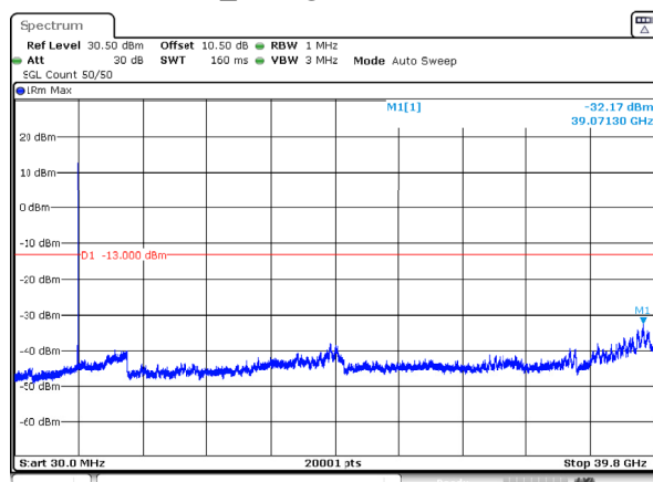
n77_3_60MHz_30kHz_3950MHz_DFT-s-OFDM QPSK_RB1@161 -32.17dBm
